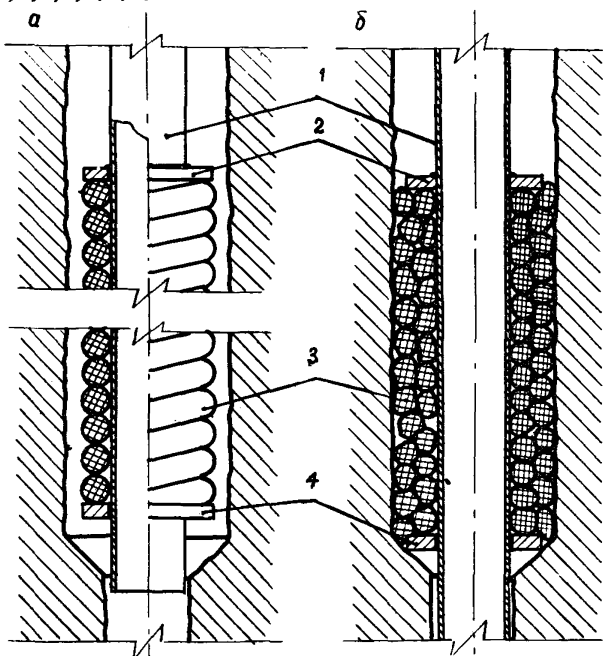
Рис. 2. Конструкция сальникового тампона при спуске в скважину (а) и в сжатом состоянии (б): 1 - об- садная труба; 2 - верхнее кольцо; 3 - сальниковая веревка; 4 - нижнее кольцо
