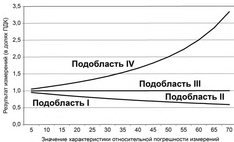
Рисунок 1 — Разбиение области возможных значений концентрации загрязняющего вещества на подобласти: I — C < (ПДК-\Delta) , II — (ПДК-\Delta) < C \leq ПДК , III — (ПДК+\Delta) < C > ПДК , IV — C > (ПДК+\Delta)
