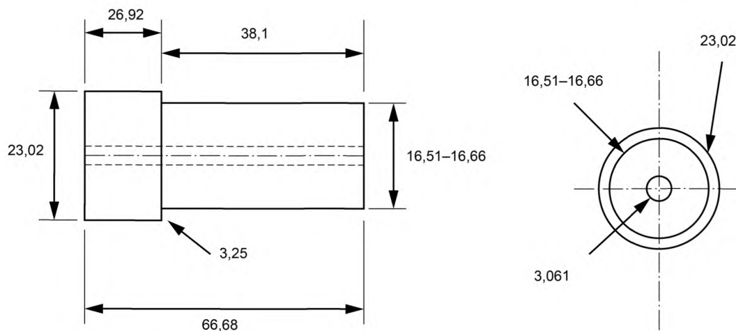
Рисунок 1 — Центрирующее устройство для центровки иглы
