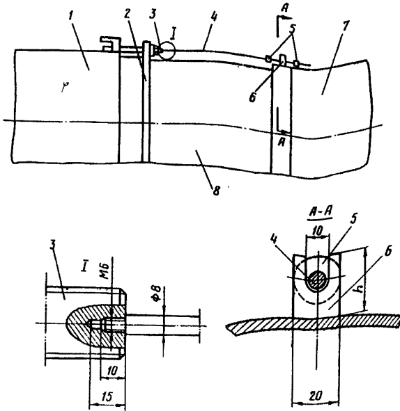
Рис.3. Фиксатор перемещения для измерения максимального перемещения стакана сальникового компенсатора:
