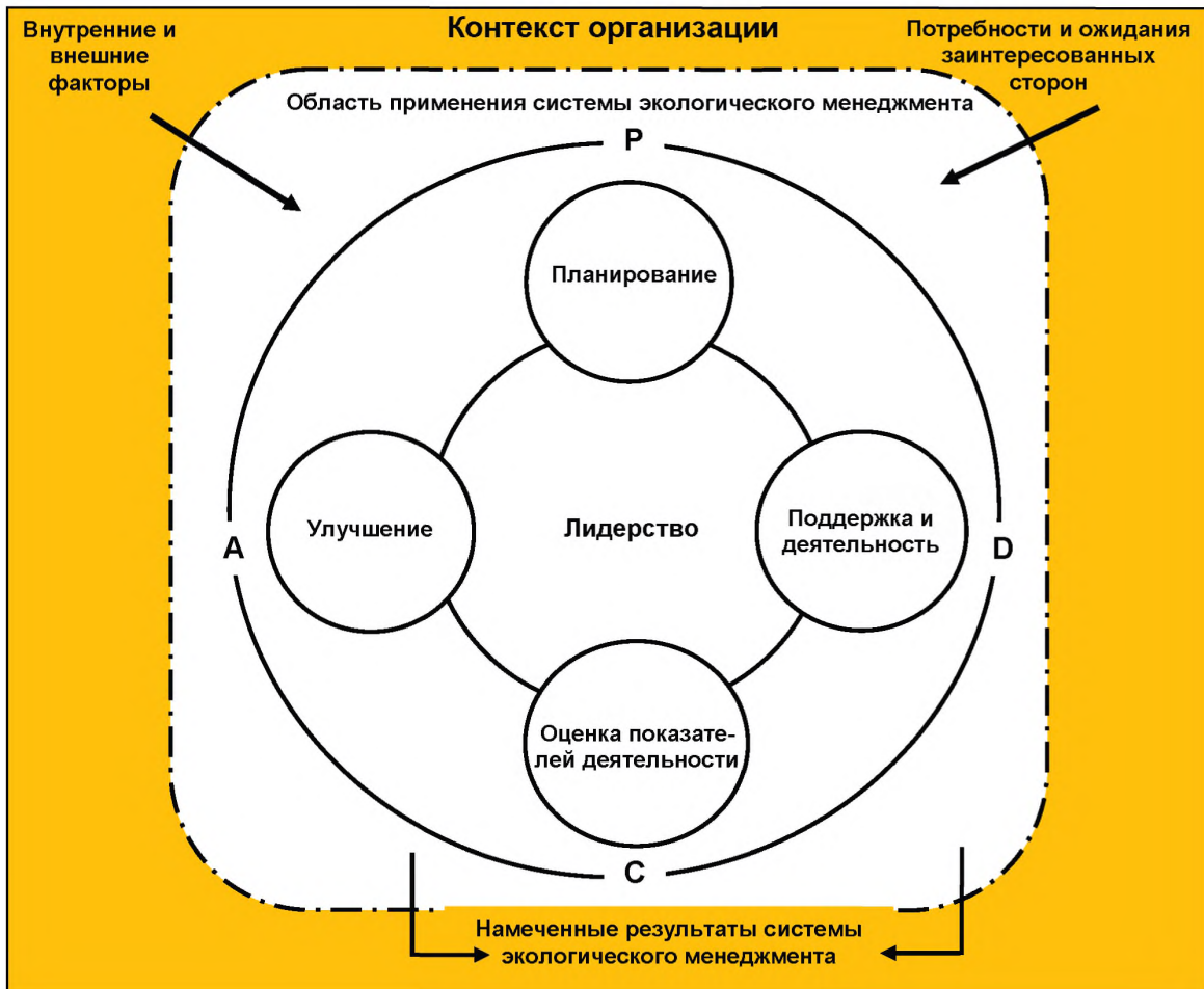
Рисунок 1 — Модель системы экологического менеджмента для настоящего стандарта
