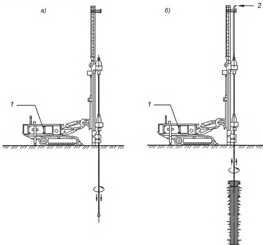
а) — бурение лидерной скважины до отметки низа элемента (прямой ход); б) — устройство грунтоцементного элемента (обратный ход) 1 — буровая установка; 2 — цементный раствор
