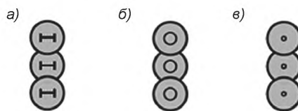
а) — двутавром; б) — трубой; в) — тремя буровыми штангами с накатанной винтовой поверхностью
