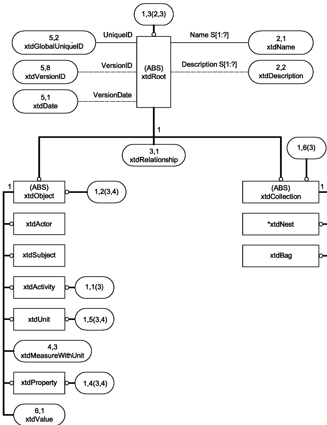
Рисунок 1 — EXPRESS-G диаграмма 1 — Верхний уровень с корневой концепцией
