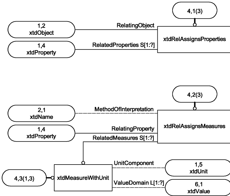
Рисунок 4 — EXPRESS-G диаграмма 4 — Назначение свойств и единиц измерений
