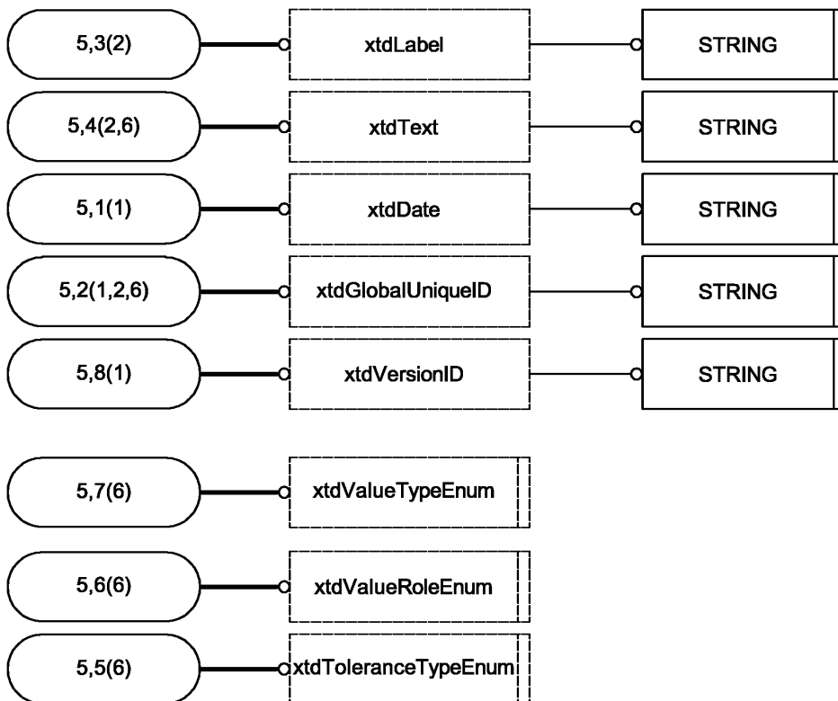
Рисунок 5 — EXPRESS-G диаграмма 5 — Основные типы
