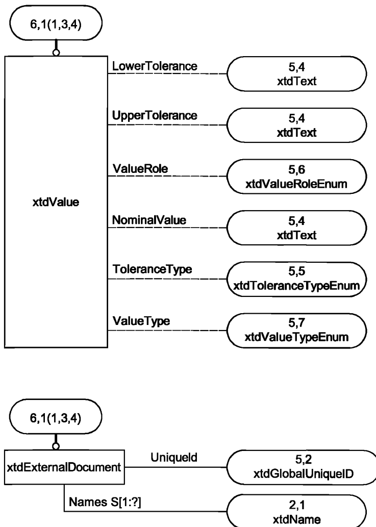
Рисунок 6 — EXPRESS-G диаграмма 6 — Значения и внешние документы
