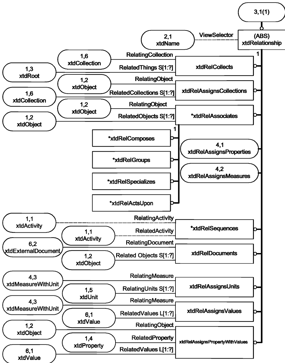
Рисунок 3 — EXPRESS-G диаграмма 3 — Отношения
