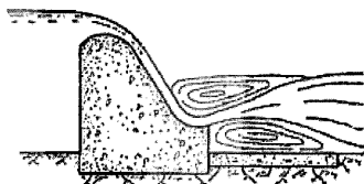
Рисунок 6 – Водосливная плотина с уступом
