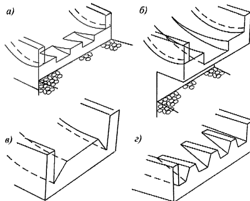
а) – зубчатый носок; б), в) – носки с направленным отбросом; г) – носок с трапециевидными расщепителями
