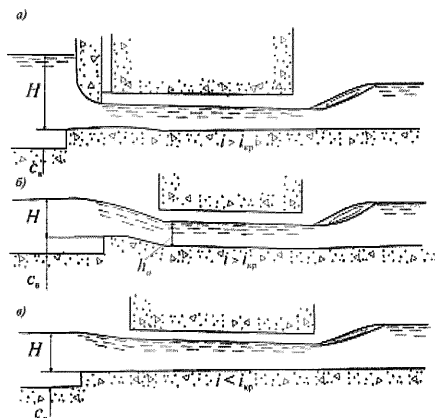
а – с забральной стенкой; б – с водосливным порогом; в – в виде водослива без порога
