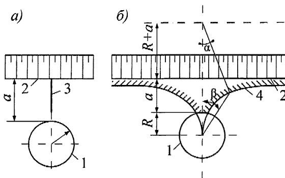
а) – при расстоянии от гребня воронки до основания откоса 3R \geq a > 2R ; б) – при 2R \geq a \geq R ; 1 – гребень воронки; 2 – основание берегового откоса; 3 – противоворотная прямолинейная стенка; 4 – противоворотная стенка криволинейного очертания
