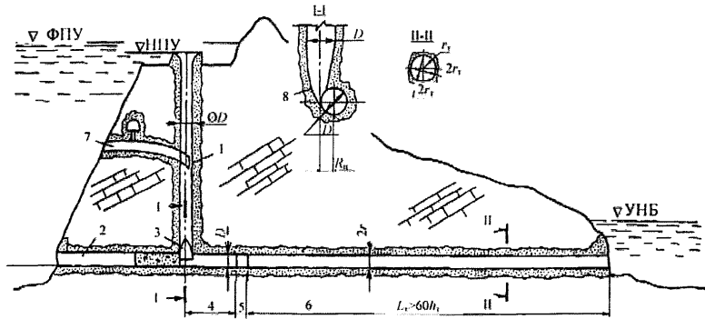
1 – шахта; 2 – строительный туннель; 3 – тангенциальный завихритель; 4 – туннель круглого сечения; 5 – переходной участок; 6 – отводящий туннель; 7 – глубинный водоприемник; 8 – цилиндрическая вставка завихрителя
