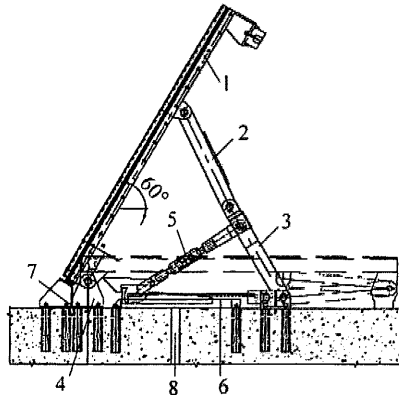
Рисунок 47 – Схематический разрез автоматического вододействующего затвора многогоразового действия
