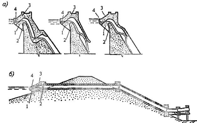
1 – входное отверстие; 2 – гребень; 3 – капор; 4 – воздухоподводящее отверстие Рисунок 31 – Типы сифонных водосбросов в теле бетонных плотин (а) и в теле грунтовой плотины (б)
