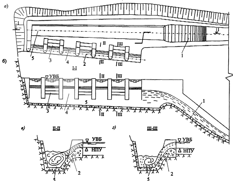
а) – план; б) – вид на боковой водослив со стороны водосбросной траншеи; е) и з) – поперечные разрезы по пролетам бокового водослива, соответственно, с носками и без носков на сливной грани; 1 – быстроток; 2 – боковой водослив; 3 – пролеты бокового водослива с носками на сливной грани; 4 – пролеты без носков ; 5 – водосбросная траншея
