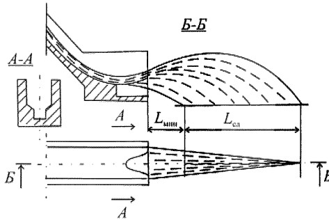
Рисунок 43 –Трамплин с фигурным вырезом
