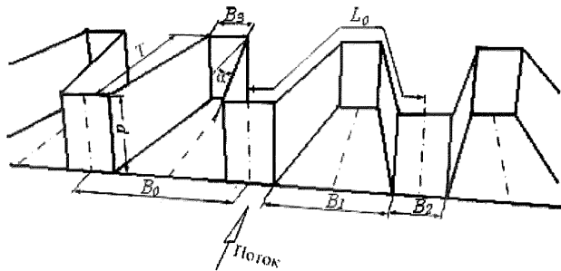
Рисунок 13 – Схема лабиринтного водослива
