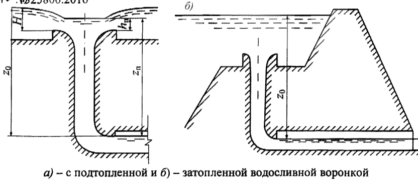
а) – с подтопленной и б) – затопленной водосливной воронкой
