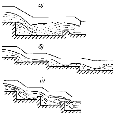
Рисунок 17 – Схемы перепадов
