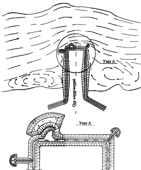
Рисунок 50 – Схема перемычки со струеотклоняющими шпорами
