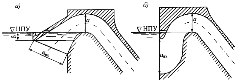
а) – прямолинейный входной участок; б) – криволинейный входной участок
