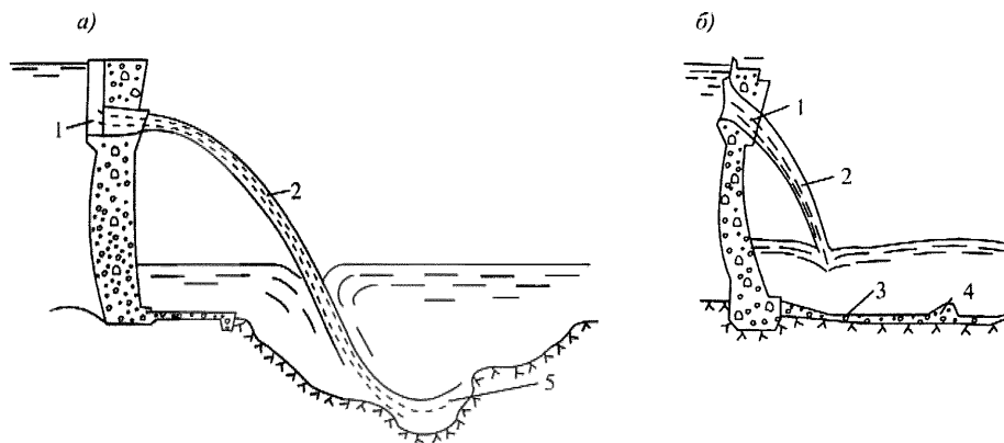
1 – глубокий водосброс; 2 – отброшенная струя; 3 – бетонное крепление; 4 – гаситель; 5 – воронка размыва
