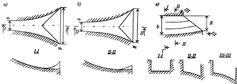
а) – симметричный рассеивающий трамплин; б) – несимметричный рассеивающий трамплин; в) – отклоняющий трамплин-вираж с косым срезом
