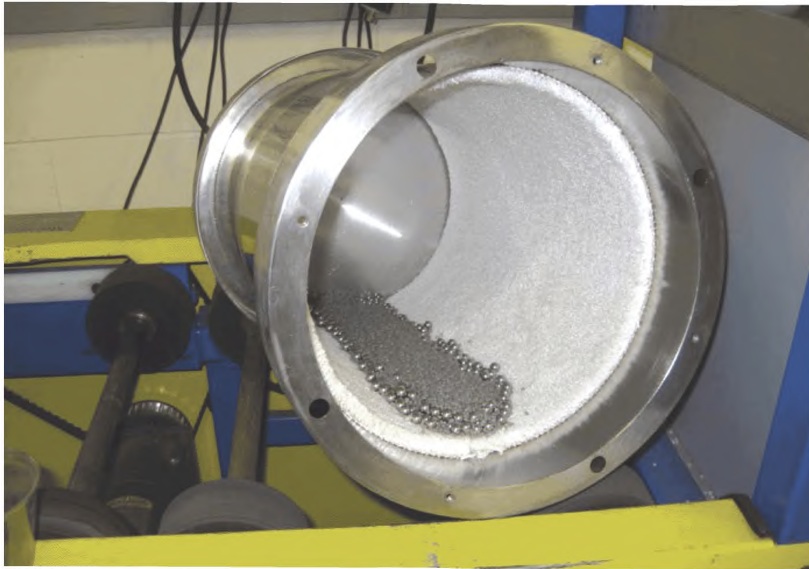
а) Цилиндр для загрязнения ковра
