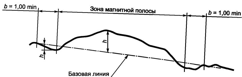
Рисунок 9 — Выпуклый профиль полосы
