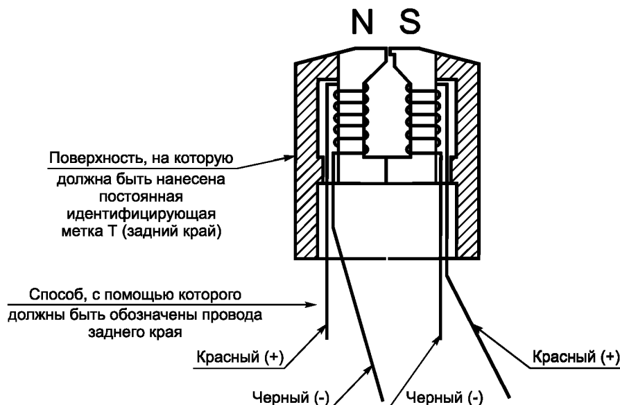
Рисунок 13 — Выводы обмоток испытательной головки записи
