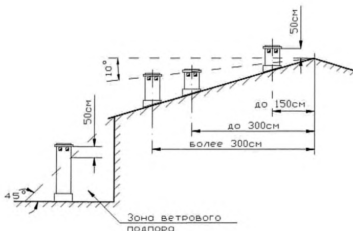
Рисунок 6.1 – Высота дымоходов в зданиях
