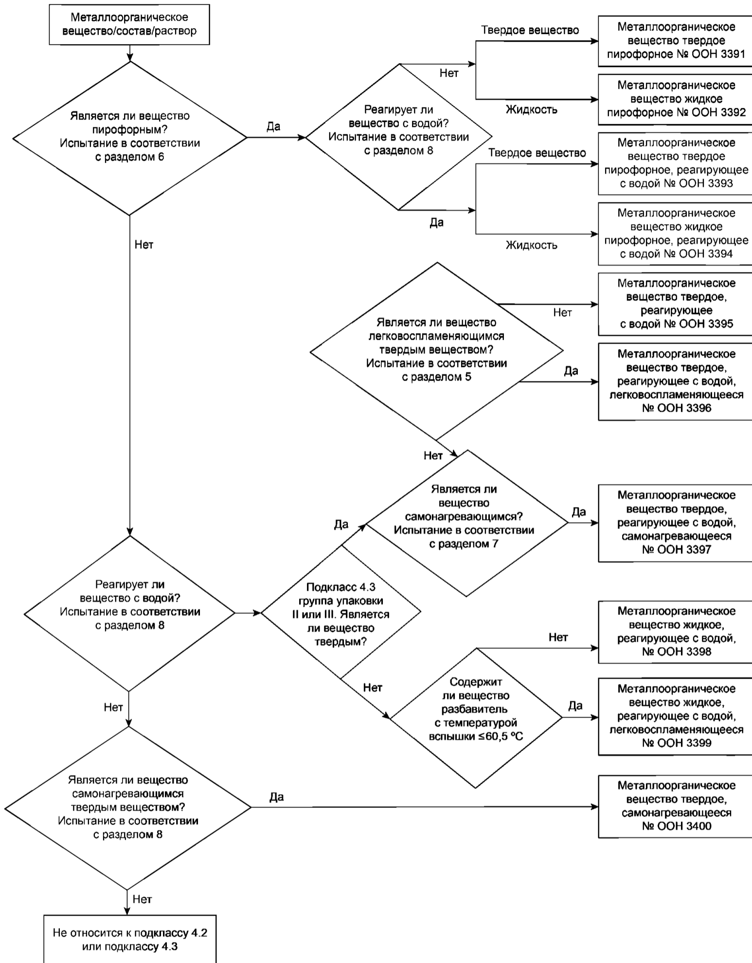
Рисунок Б.3 — Схема классификации металлоорганических веществ
