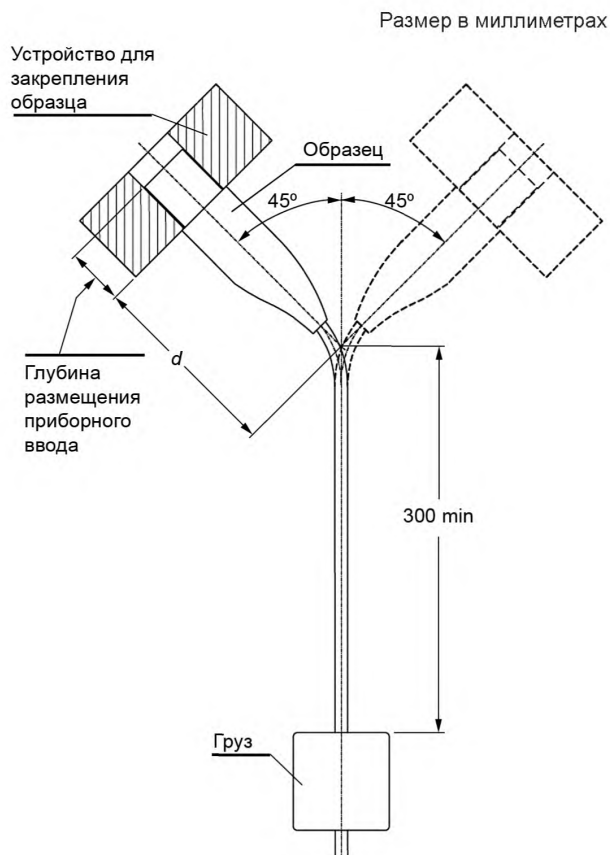
Рисунок 2 — Устройство для испытания на изгиб
