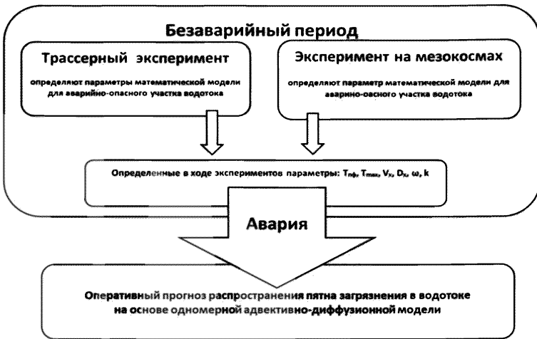
Рисунок 1 – Общая схема оперативного мониторинга аварийного загрязнения водотока
