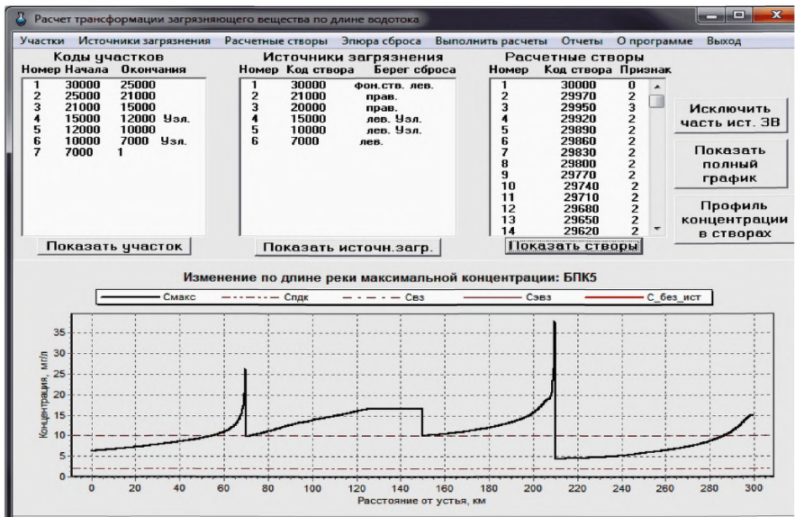
Рисунок А.12 – Главная экранная форма после завершения расчета стационарной задачи
