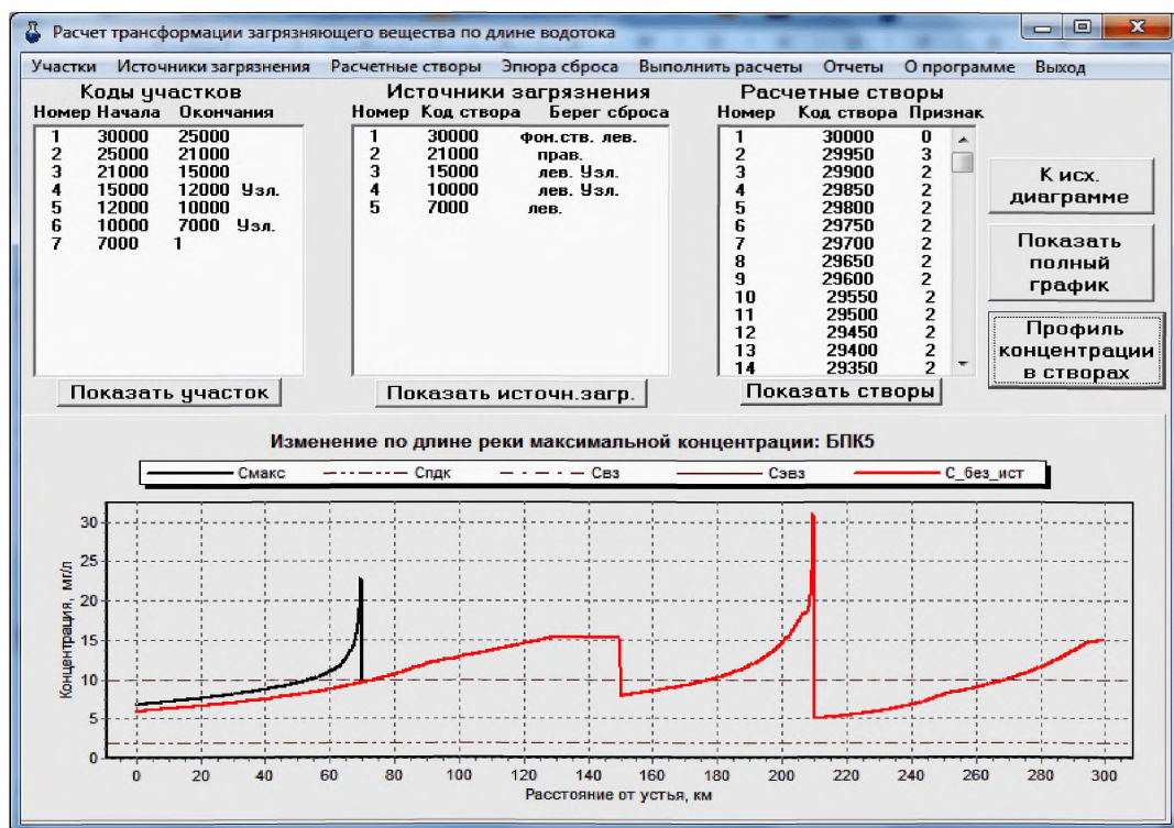
Рисунок А.16 – Пример иллюстрации результата решения подзадачи с исключением части источников ЗВ.
