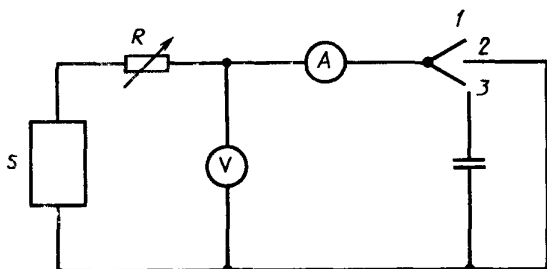
Рисунок 3 — Испытательная схема постоянного тока
