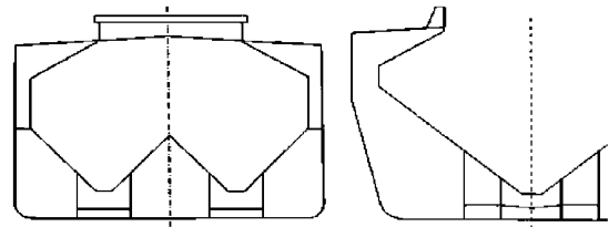
Рис. 2.2.9 Типовые сечения мидель-шпангоута саморазгружающегося навалочного судна
