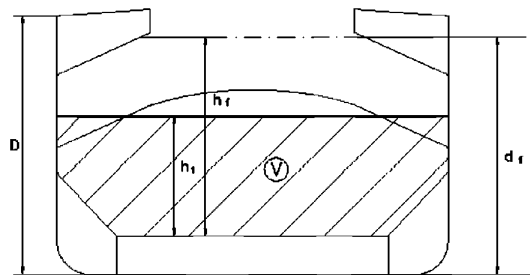
Рис. 5.10.2.2 Схема загрузленного трюма ( V — объем груза, м 3 )
