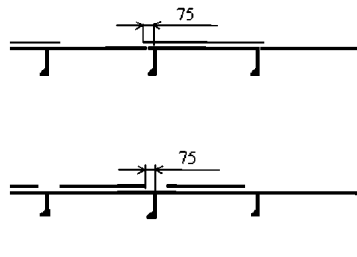
Рис. 5.2.2.5-1 Расположение накладных полос
