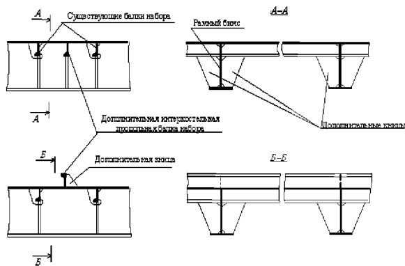
Рис. 5.2.2.5-2 Установка дополнительных балок набора
