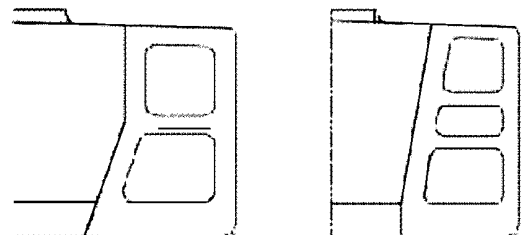
Рис. 2.2.7.2 Типовые сечения мидель-шпангоута нефтерудовоза
