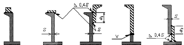
Рис. 5.2.4.1-1 Подкрепления балок набора:
