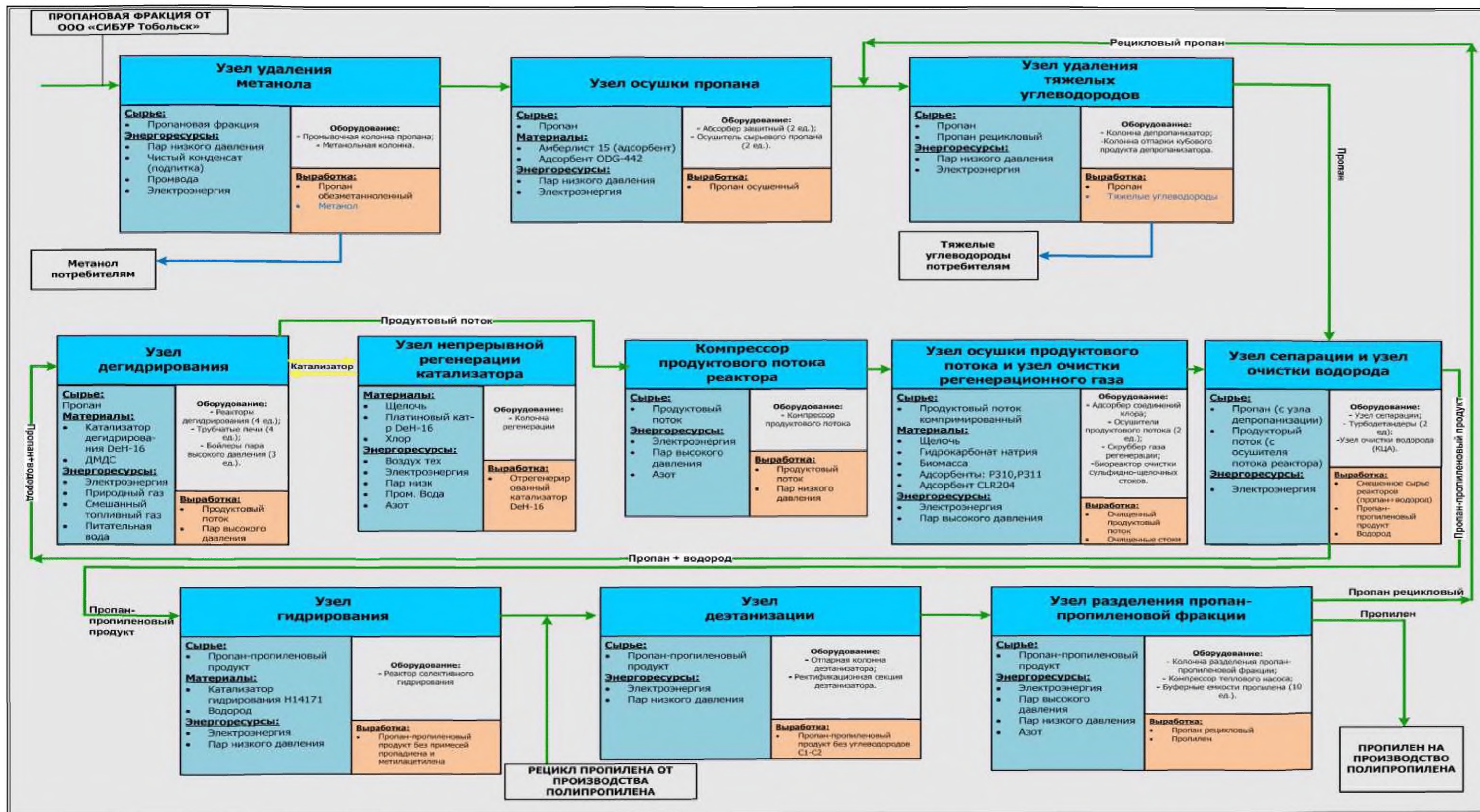
Рисунок 2.2.1 – Принципиальная технологическая схема процесса "Olefex"
