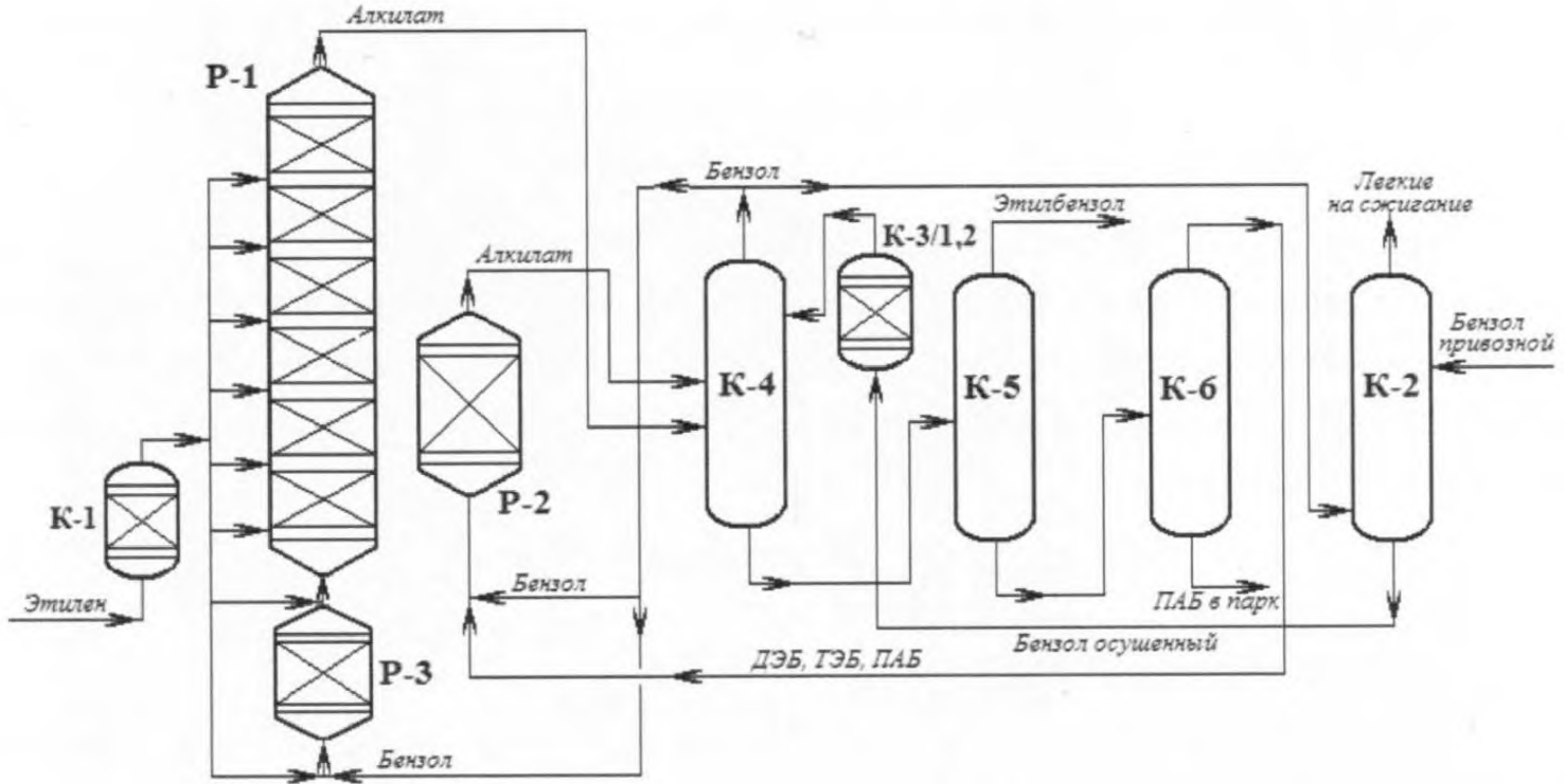
К-1, К-3/1,2 – адсорберы; P-1, P-2, P-3 – реакторы; К-2, К-4, К-5, К-6 – ректификационные колонны
