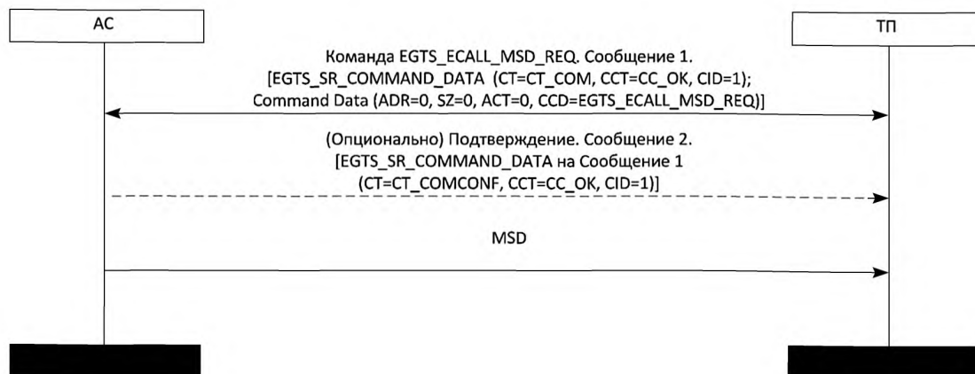
Рисунок 11 — Отправка команды EGTS_ECALL_MSD_REQ по SMS
