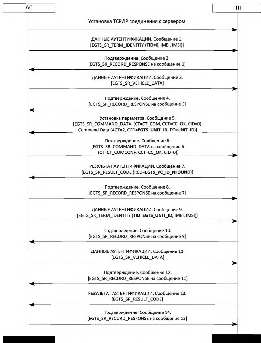
Рисунок 9 — Алгоритм конфигурации UCSB с использованием GPRS
