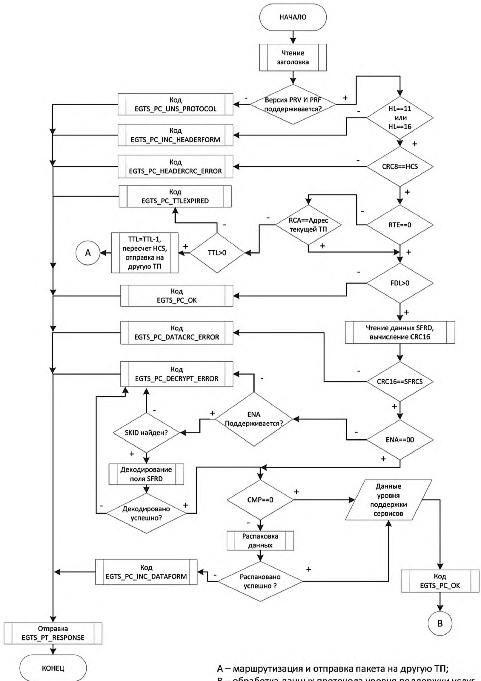
Рисунок 2 — Блок-схема алгоритма сборки пакета протокола транспортного уровня при приеме
