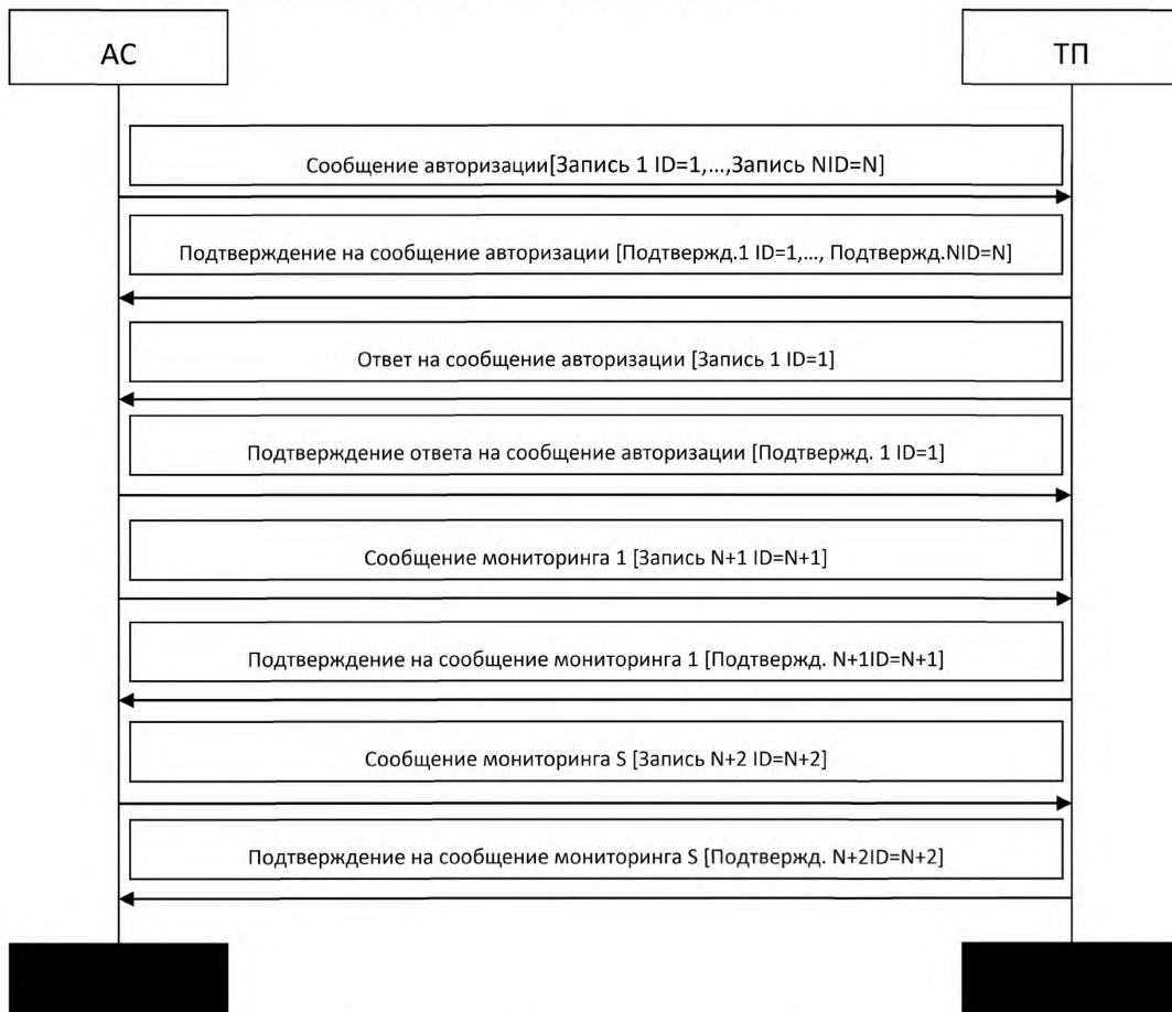
Рисунок 7 — Диаграмма обмена сообщениями
