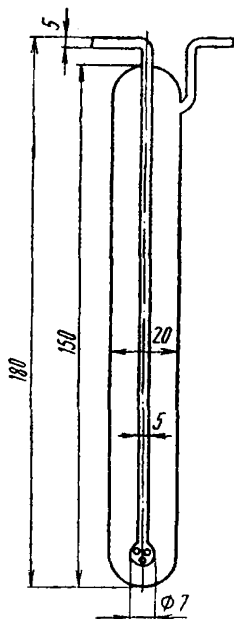
Рис. 6. Поглотительный прибор Петри
