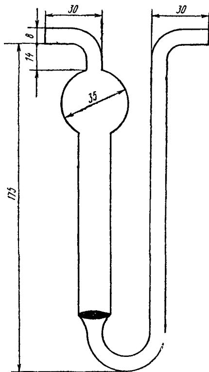
Рис. 8. Поглощительный прибор с пористой стеклянной пластинкой
