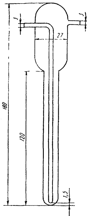
Рис. 7. Поглотительный прибор Зайцева
