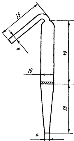
Рис. 5. Стекло́нная трубка с пористой пластинкой для отбора проб воздуха
