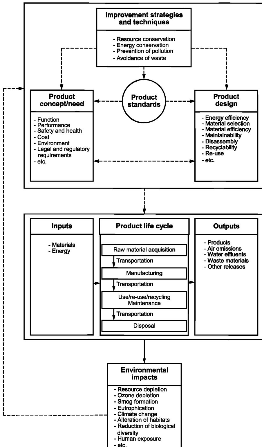
Рисунок 1 — Взаимосвязь между положениями стандартов на продукцию и экологическими аспектами и воздействиями, связанными с продукцией на протяжении ее ЖЦ
