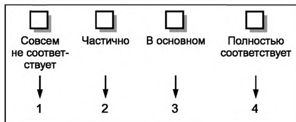
Рисунок 4 — Кодирование ответов
