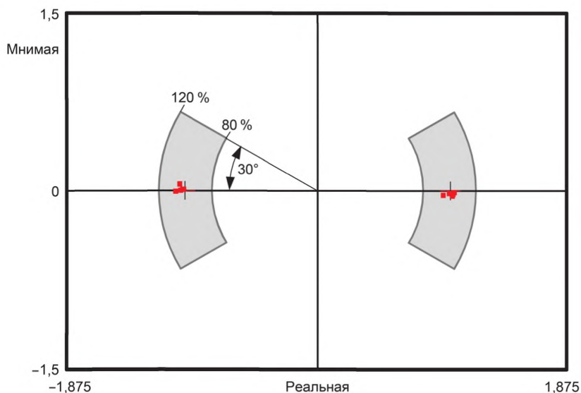
Рисунок 3 — Совокупная диаграмма и границы измерений для BPSK-модуляции
