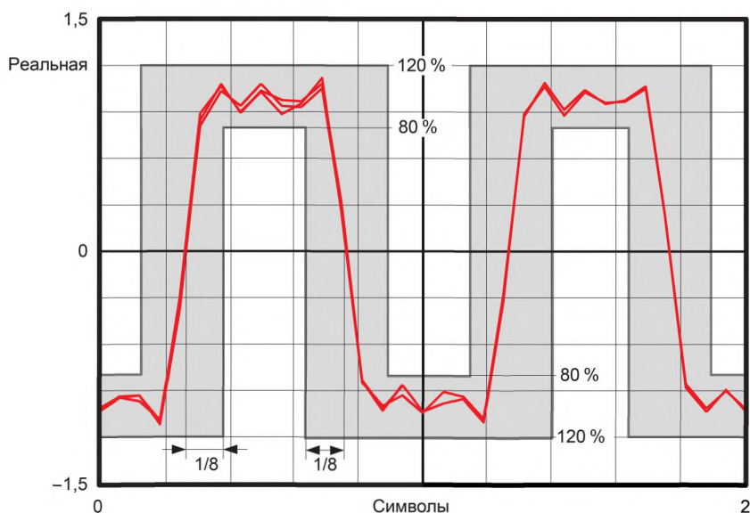
Рисунок 4 — Индикаторная диаграмма и границы измерений для BPSK-модуляции
