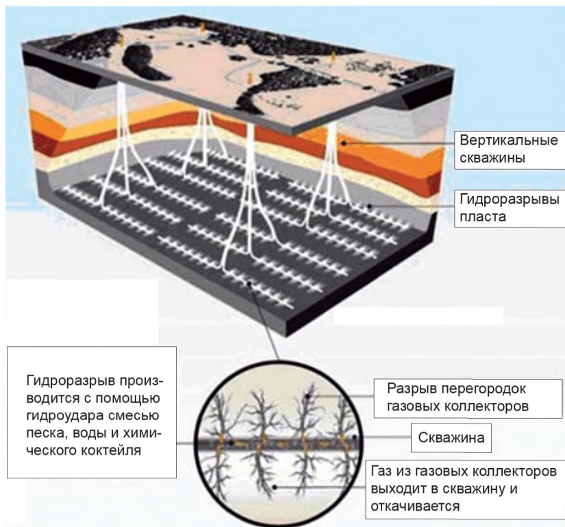
Рисунок 4 — Бурение одноствольных и многоствольных горизонтальных скважин с последующим использованием гидроразрыва пласта
