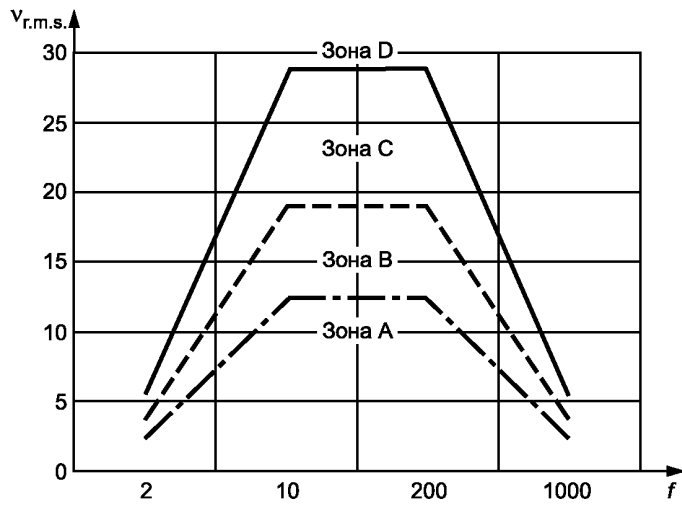
Рисунок В.10 — Границы зон для вибрации трубопроводов и гасителей пульсаций компрессора с вертикальным расположением цилиндров
