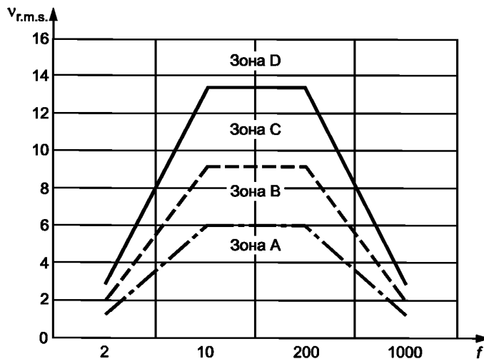
Рисунок С.2 — Границы зон направляющих крейцкопфа
