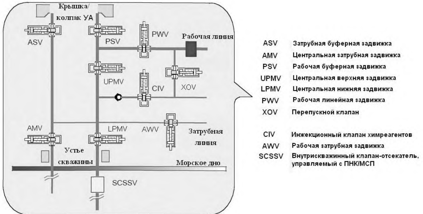
Рис. 1 Типовой комплект оборудования и арматуры
