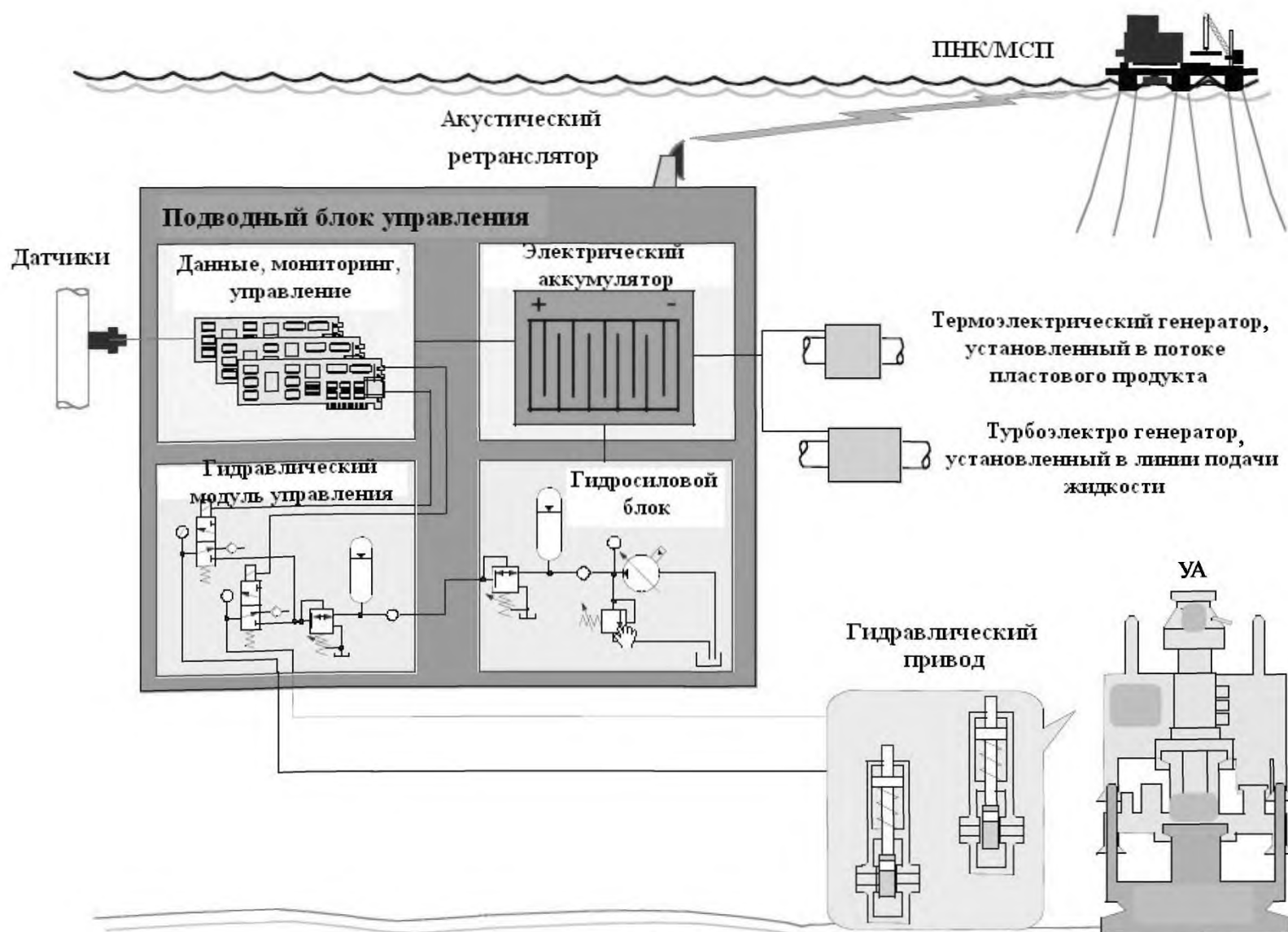
Рис. 7 Автономные системы (SPARCS)
