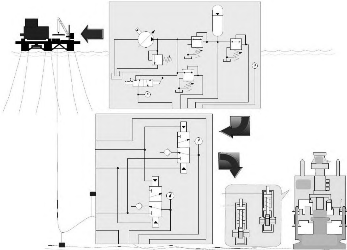
Рис. 4 Гидравлические системы с последовательным управлением
