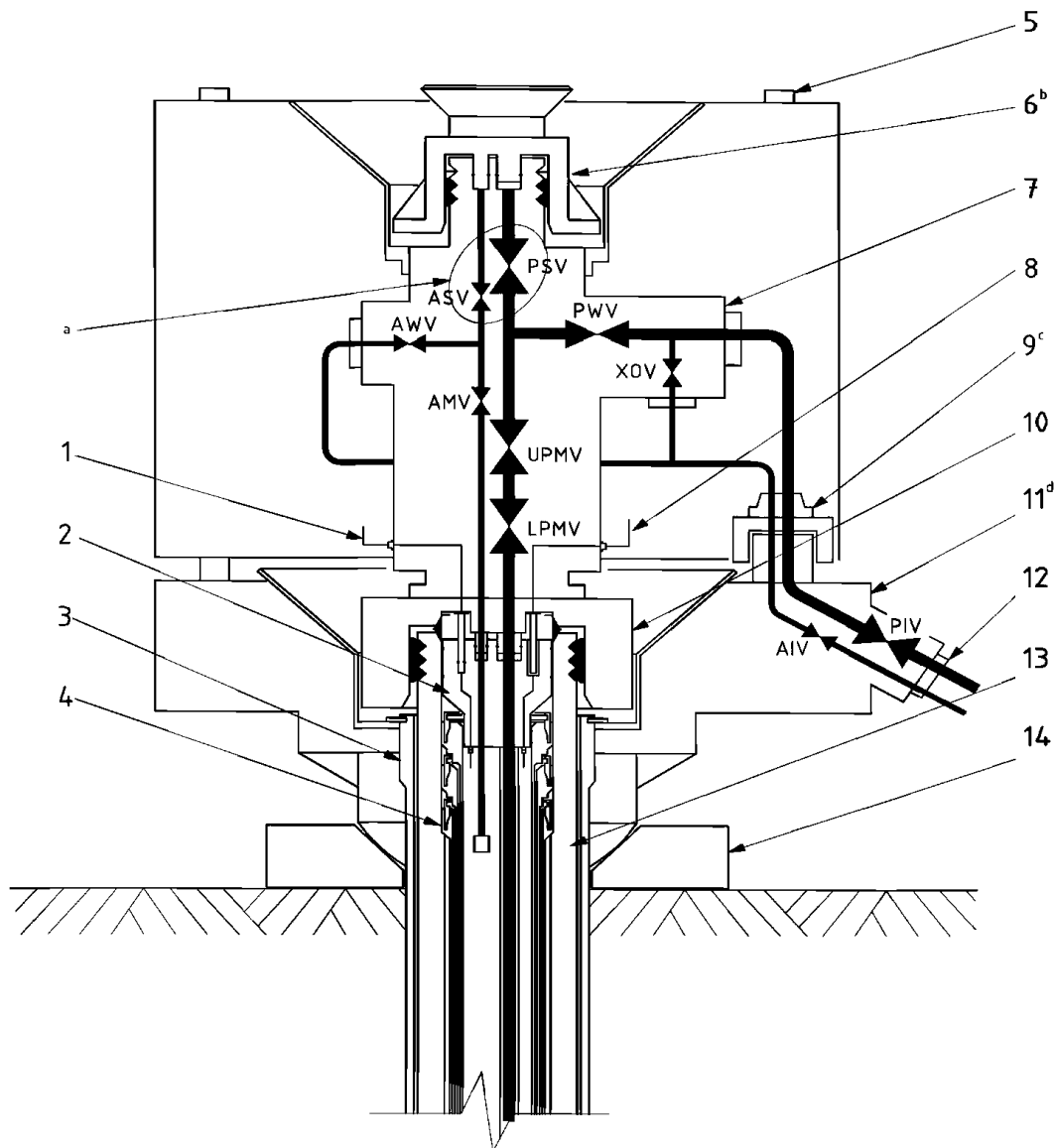
Рис. 1 Вертикальная устьевая арматура (VXT)
