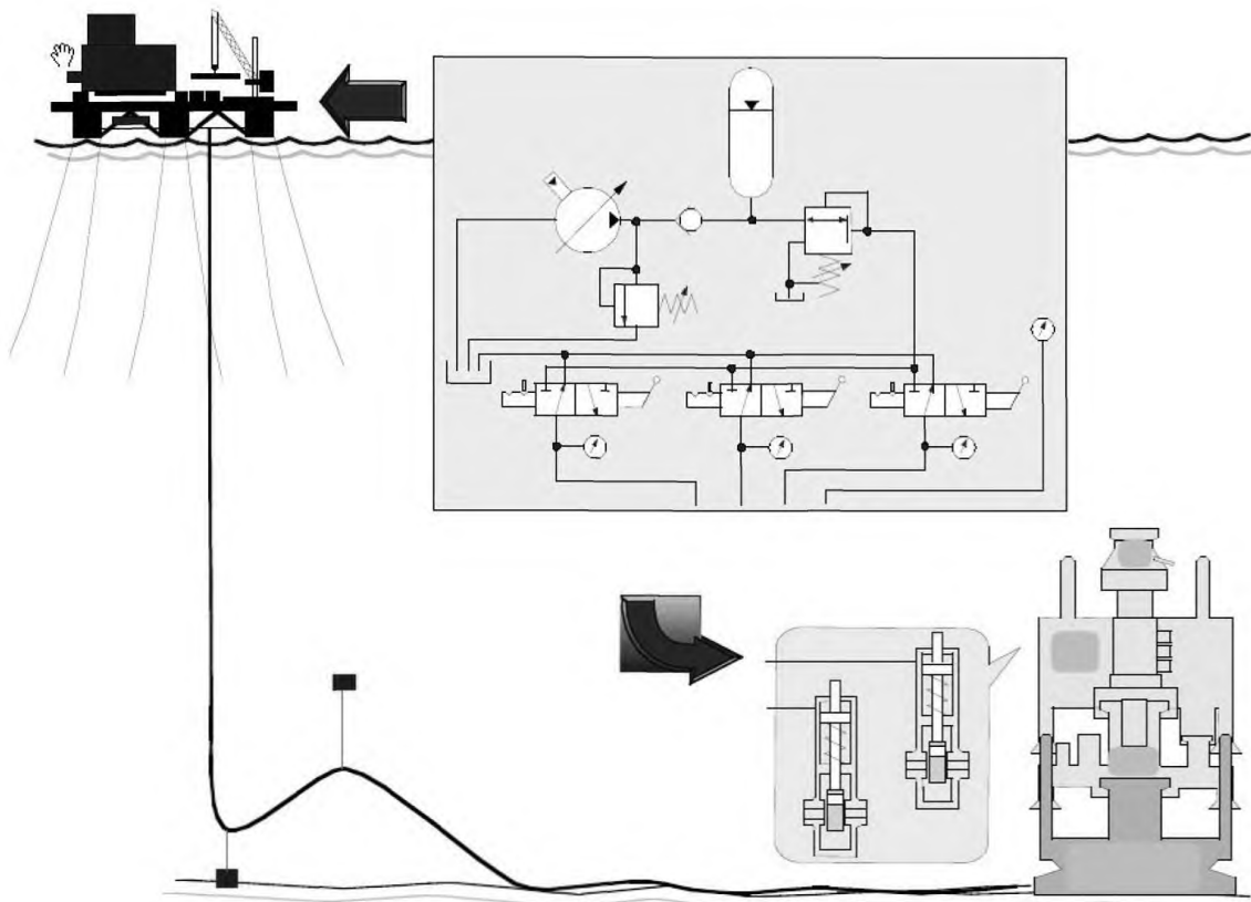
Рис. 2 Гидравлические системы с непосредственным гидроприводом
