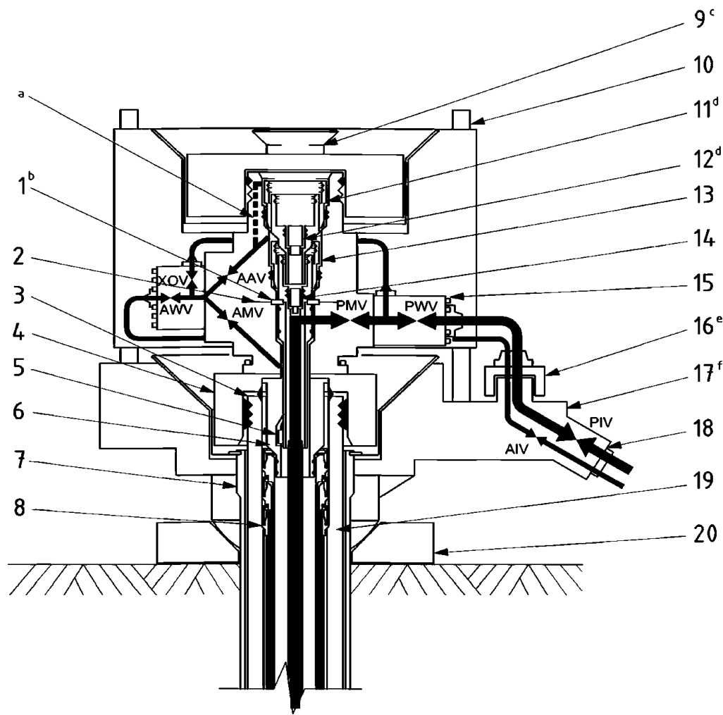
Рис. 5 Горизонтальная устьевая арматура (НХТ)
