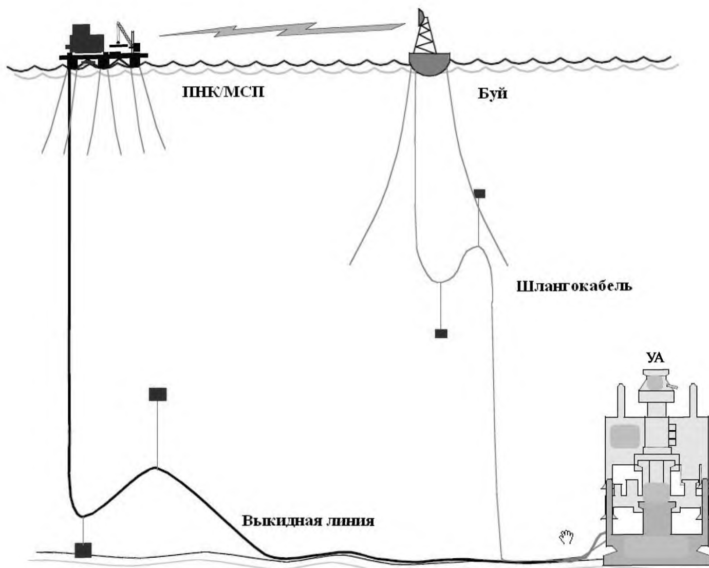
Рис. 8 Интегрированные буи контроля и управления (ICB)
