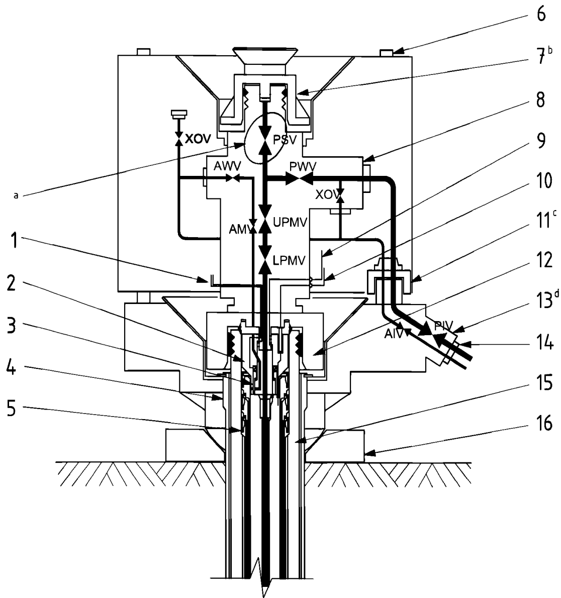
Рис. 3 Вертикальная устьевая арматура (VXT) концентрического типа
