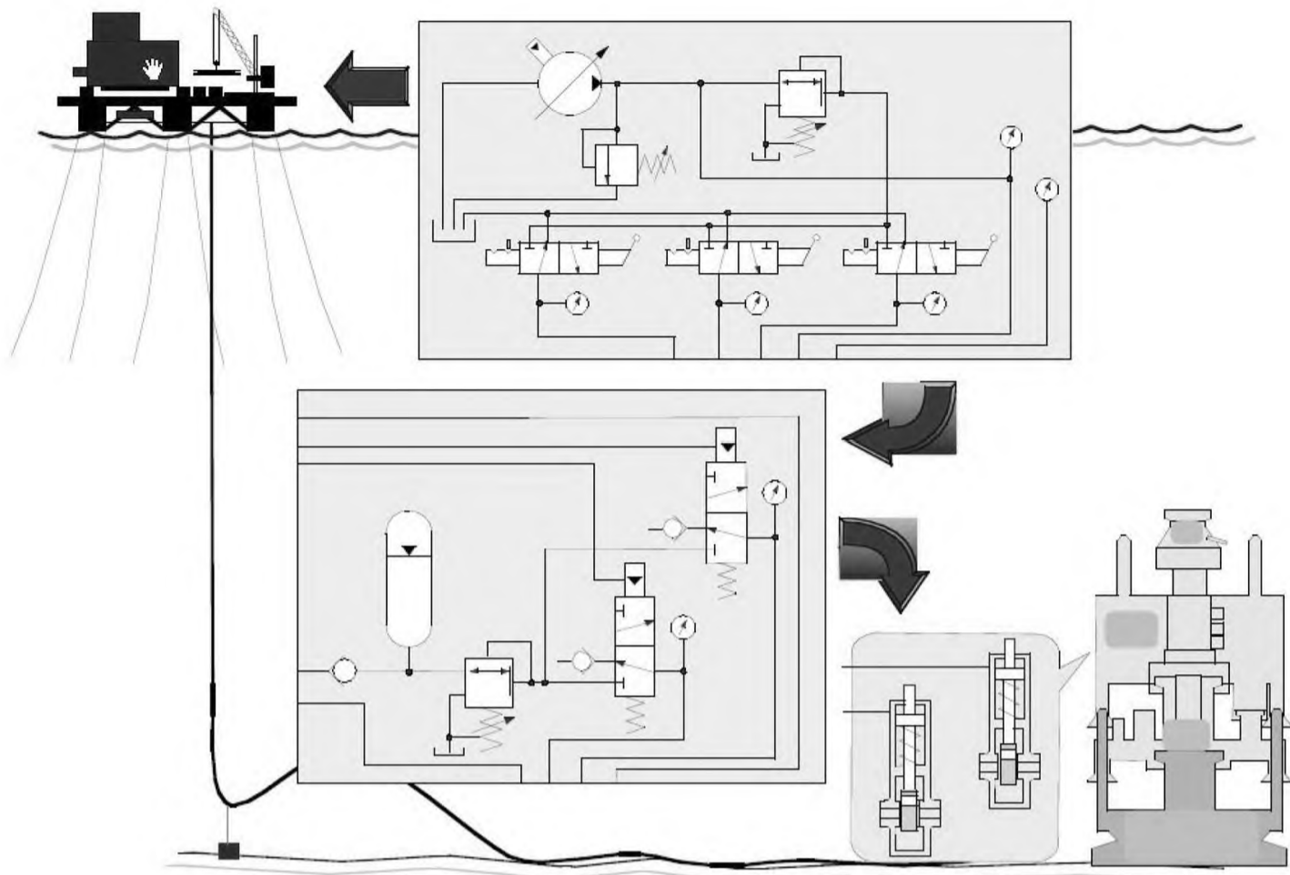
Рис. 3 Гидравлические системы с подводным управляющим модулем
