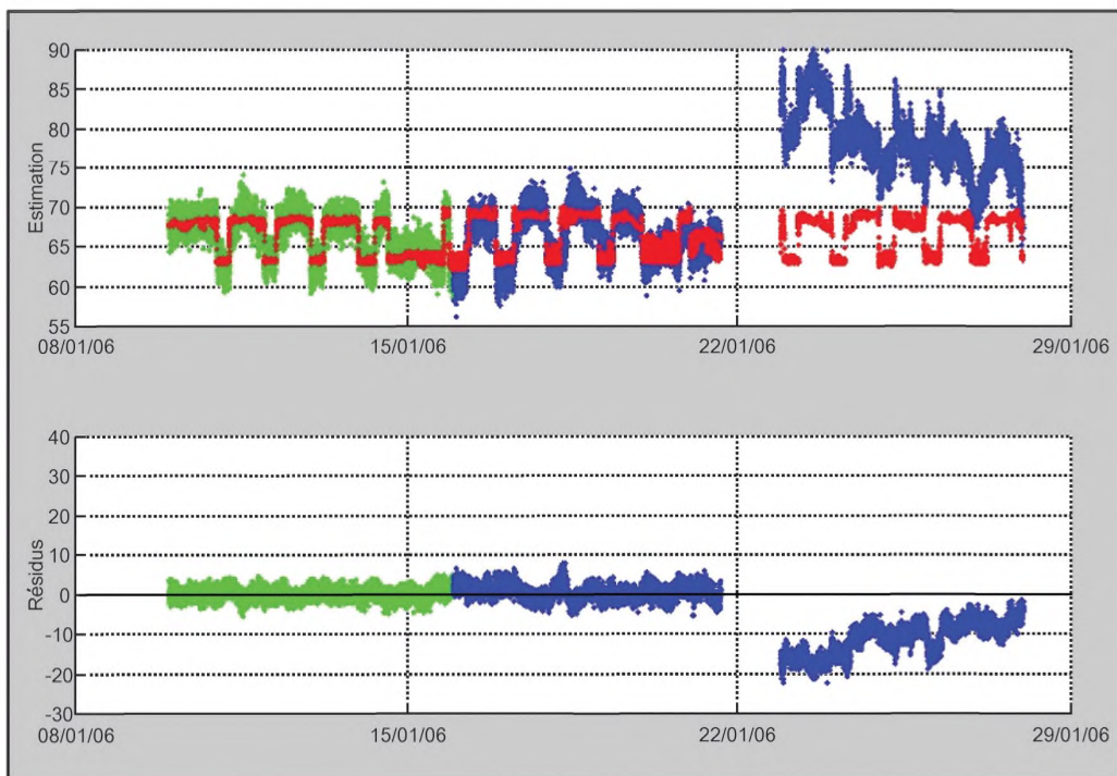
Рисунок 1 — Контроль перемещений вала газовой турбины
