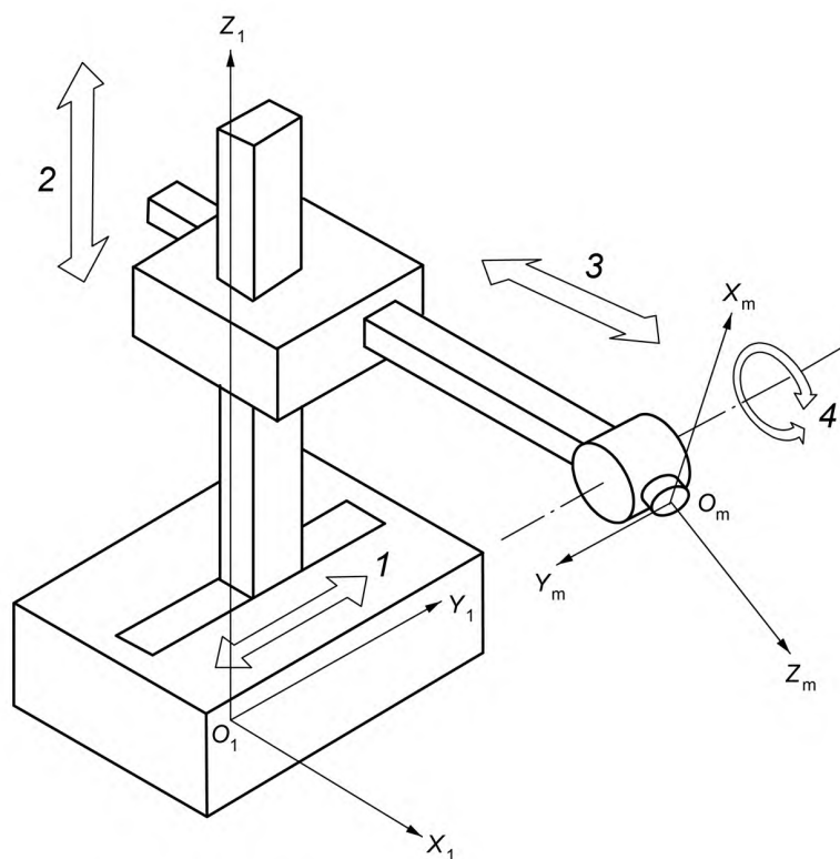
Рисунок А.1 — Робот с прямоугольной системой координат
