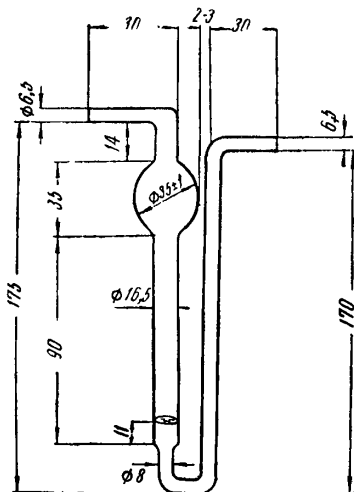
Рис. 6. Поглотительный прибор с пористой пластинкой
