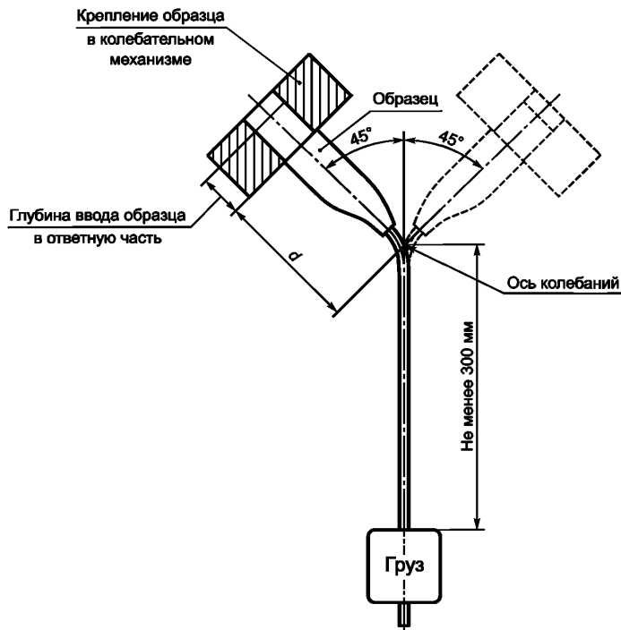
Рисунок 2 — Схема перемещения испытуемого образца неразъемного соединителя во время испытания прочности на изгиб
