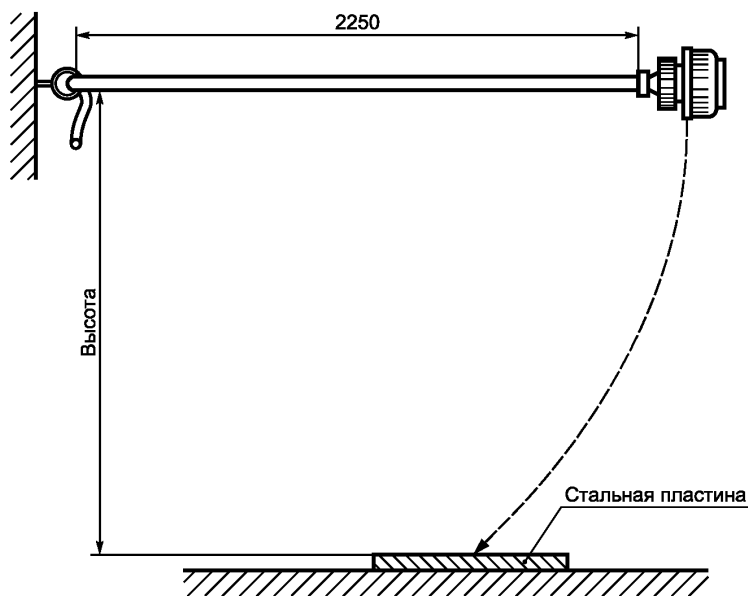
Рисунок 1 — Пример монтажа соединителя
