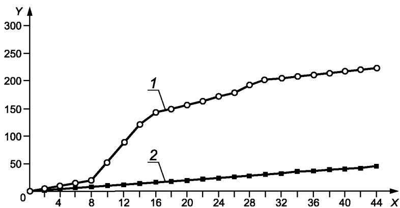
Рисунок В.1 — Кривая выделения диоксида углерода
