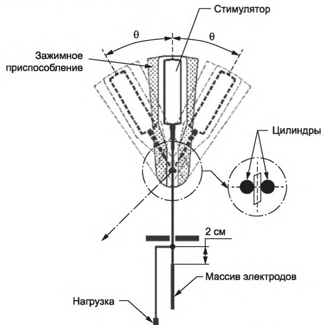
Рисунок 105 — Испытательный стенд сгибания
