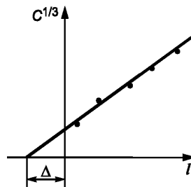
Рисунок 7 — Схема определения поправки |\Delta|
