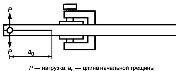
Рисунок 6 — Схема подращивания трещины по методу А
