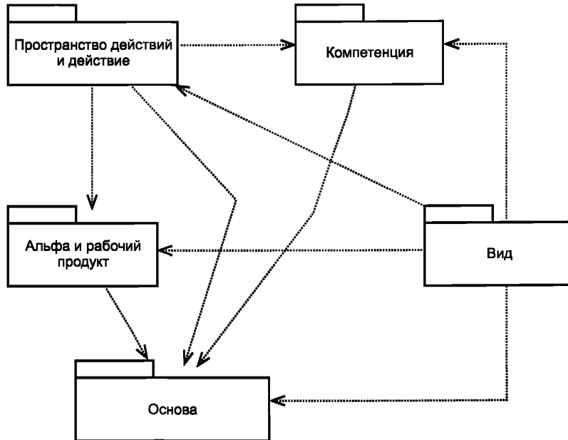
Рисунок 2 — Модель языка
