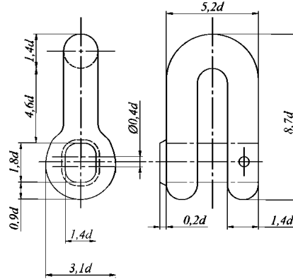
Рис. 7.1.3-6 Концевая скоба
