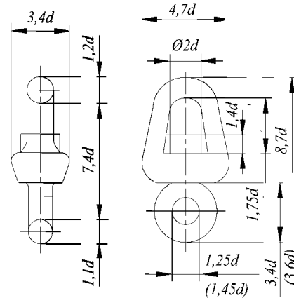
Рис. 7.1.3-7 Вертлюг
