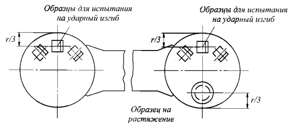
Рис. 7.2.3.2.6.1 Расположение образцов. Звено цепи
