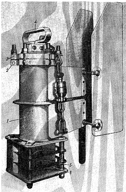
Рис.12.5 Измеритель течений БПВ-2
