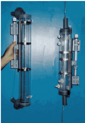
Рис. 7.6. Модель Clear Water Sampler .
