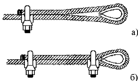
Рис. 6.80 Постановка тросовых зажимов
