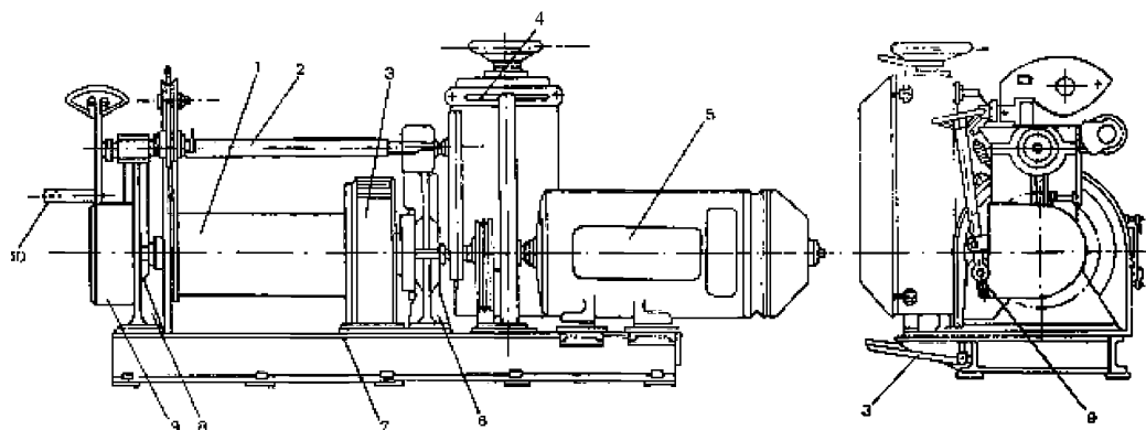
Рис. 6.75 Лебедка ЛЭРОК
