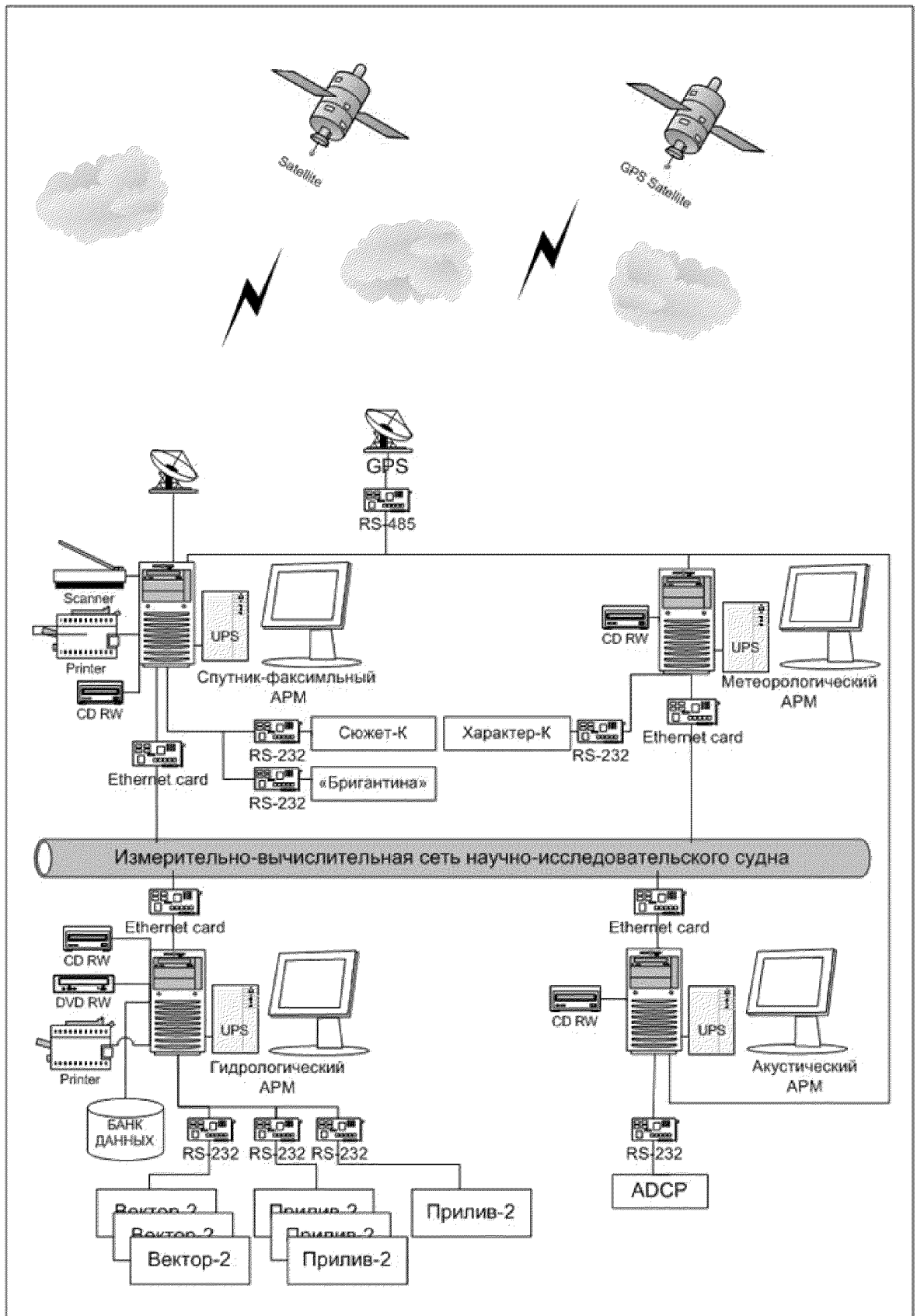
Рис.19.1 Состав ИВС научно-исследовательского судна
