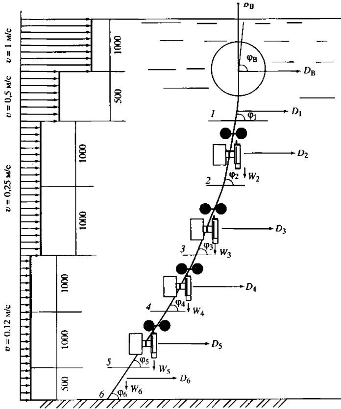
Рис. 17.6 Схема гидродинамического расчета нагрузок на буйреп притопленной АБС
