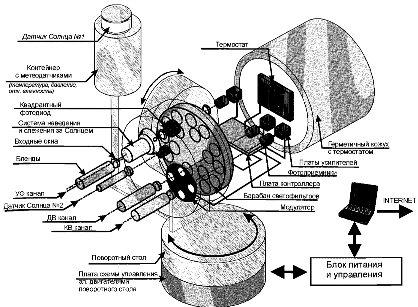
Рис.15.9 Устройство солнечного фотометра SP-6
