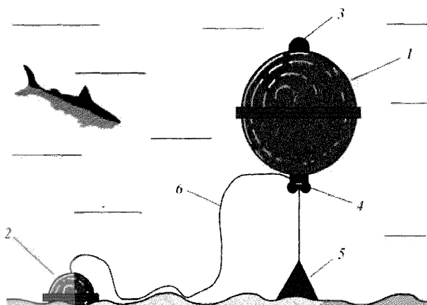
Рис. 1.1 Сейсмическая донная станция (ИО РАН): 1 - основной блок электроники; 2 - блок сейсмоприемников; 3 - гидроакустическая антенна размыкателя; 4 - механизм размыкателя; 5 - якорь-груз; 6 - гибкий кабель-трос
