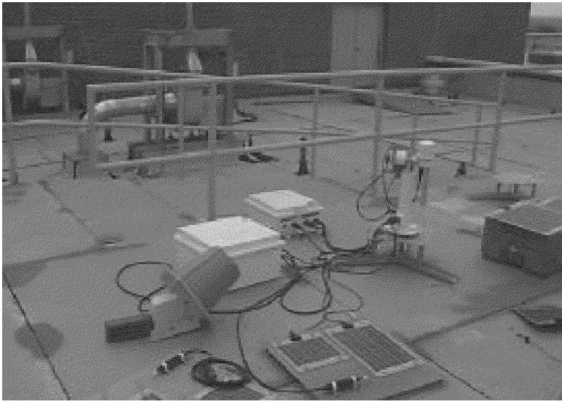
Рис.15.5 а) Прибор CIMEL
