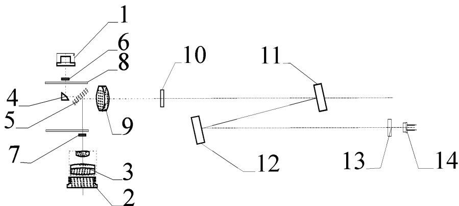
Рис.14.2 Оптическая схема судового измерителя яркости моря.
