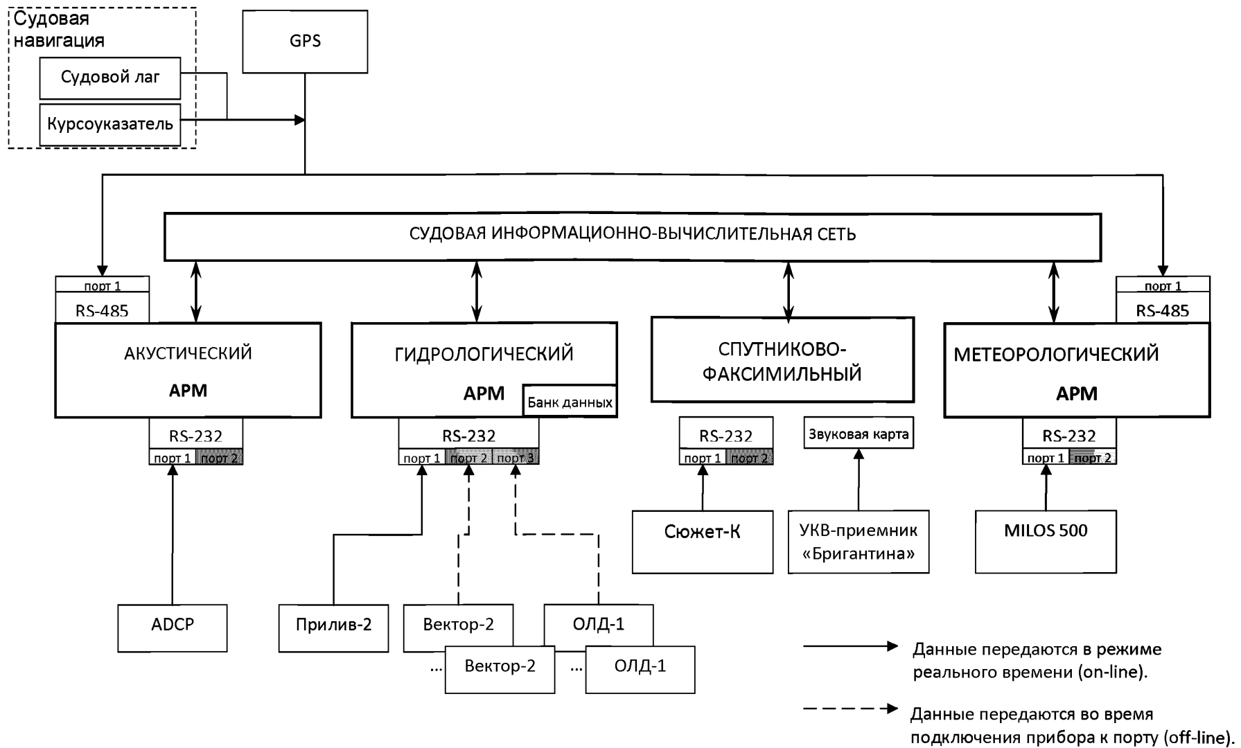
Рис. 19.2 Структура ИВС научно-исследовательского судна.
