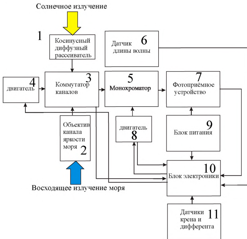
Рис.14.1 Блок схема судового измерителя яркости моря
