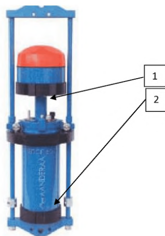
Рис.9.5 Профилометры RDCP 600. 1 - доплеровский радар, 2 - корпус
