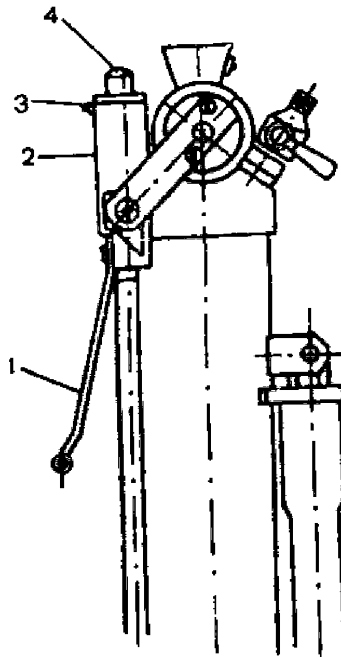
Рис. 7.15 Спускной механизм морского батометра.
