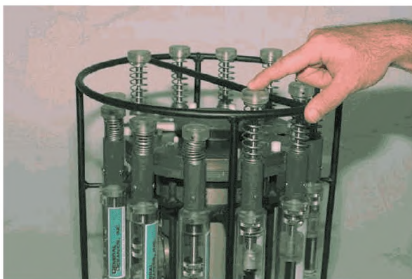
Рис. 7.12 Модель 1014 Syringe Sampler System , клапаны доступа воды в батометры.
