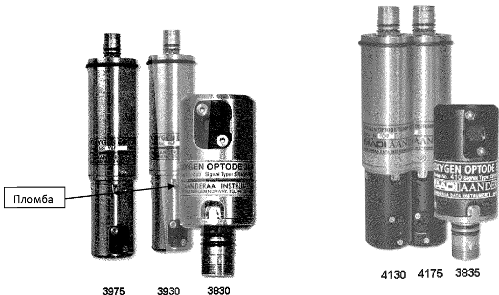
Рис.16.16 Общий вид датчиков
