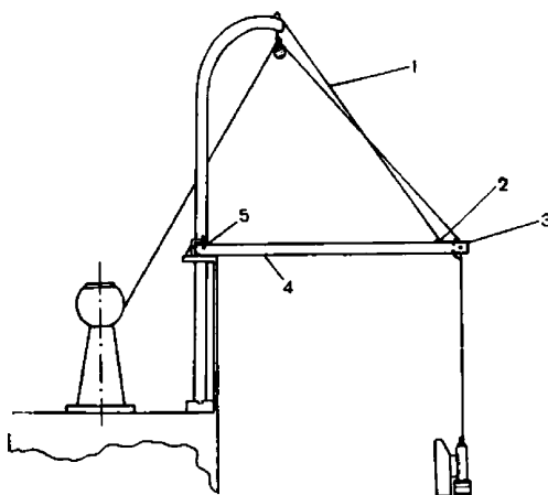
Рис. 6.76 Выстрел
