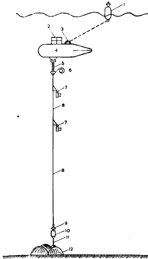
Рис. 17.7 Схема станции с притопленным буюм для больших глубин.
