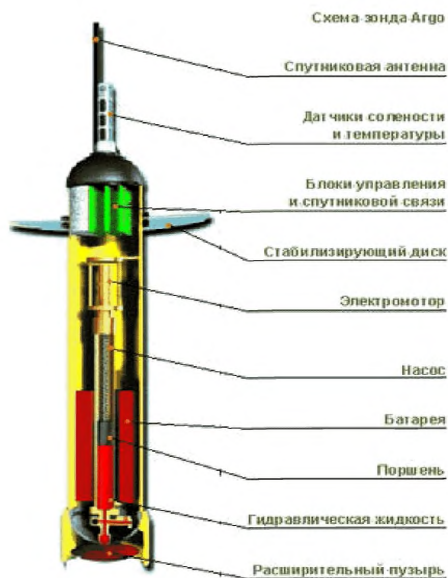
Рис.9.3 Схема зонда Argo
