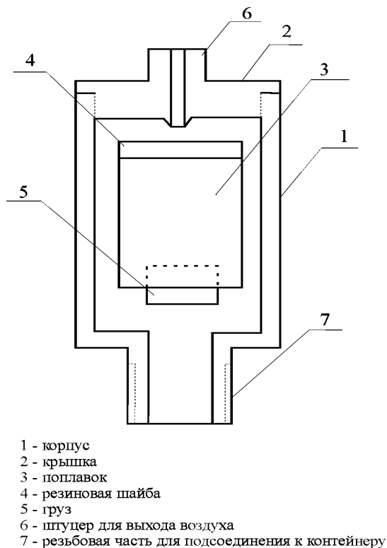
Рис.16.11 Автоматический воздушный клапан
