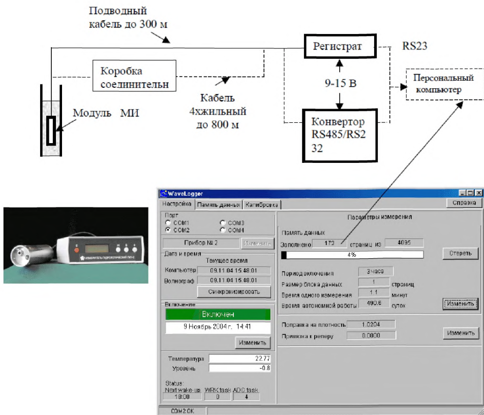
Рис.13.1 Вариант применения прибора с отображением получаемой информации на ПИ, записью в память регистратора ПИ и последующим считыванием в персональный компьютер. Внизу в левом углу рисунка изображен прибор ГМУ-2, состоящий из МИ (цилиндр) и РИ (прямоугольная коробка)
