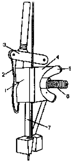
Рис. 7.14. Зажимное устройство морского батометра
