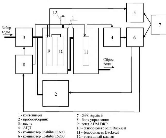
Рис. 16.10 Схема измерительной установки
