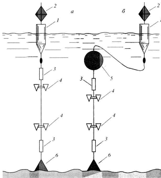
Рис. 17.1 Примеры автономных буйковых станций с поверхностным буюм (а) и станции с несущим притопленным и маркировочным поверхностным буюм (б): 1 – поверхностный цилиндрический буй; 2 – уголкоый отражатель; 3 – измеритель течений и температуры; 4 – седиментационная ловушка; 5 – притопленный буй; 6 – якорь-груз.
