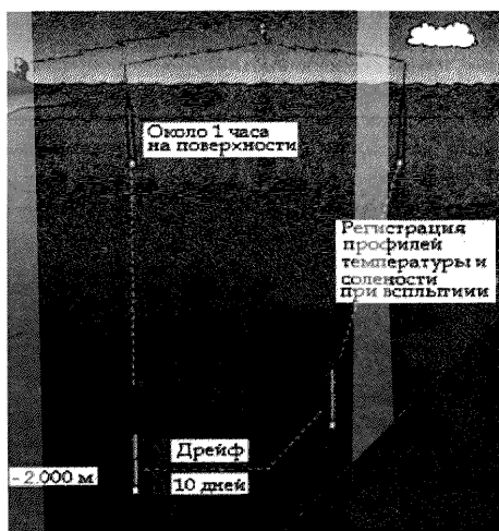
Рис.1.2 Схема работы буя-профилемера программы АРГО
