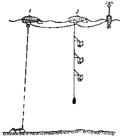
Рис. 17.4 Схема буйковой станции для средних глубин. 1,2—поддерживающие буй
