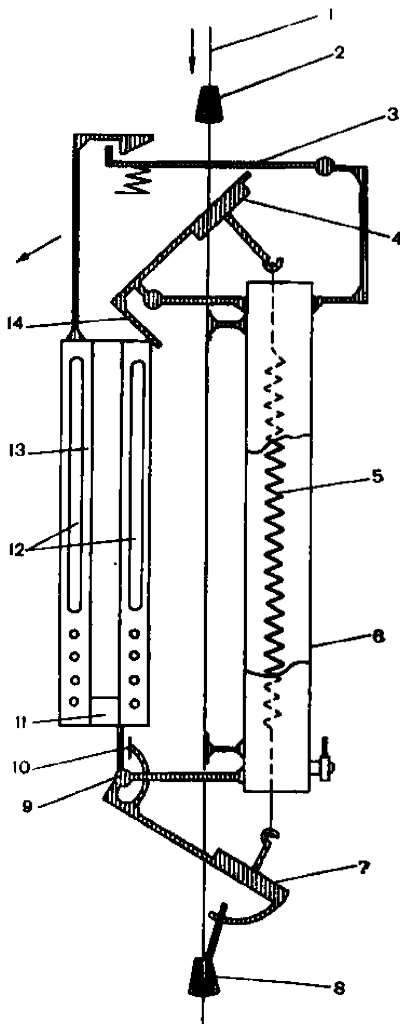
Рис. 7.17 Схема морского батометра ААНИИ
