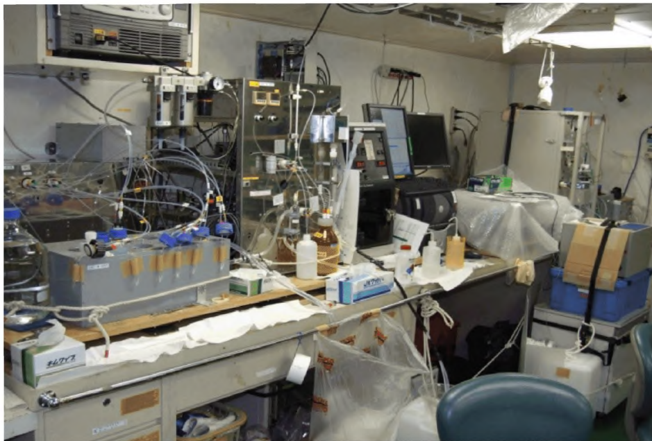
Рис.6.6 Пример интерьера лаборатории на японском RV Mirai. На снимке представлен современный комплекс по определению в пробах воды большого ряда химических элементов. В верхней левой части рисунка виден мощный кондиционер, стабилизирующий температуру в помещении. Комплекс нуждается в стабилизированном электропитании. Поручень, идущий вдоль крышки стола, следует признать удачным конструктивным решением. Наличие такого поручня способствует успешной работе оператора химического комплекса в качку.
