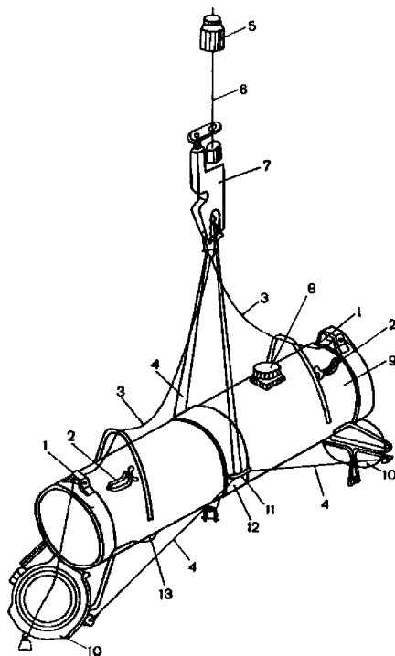
Рис. 7.19 Батометр ГМ-42 большого объема:
