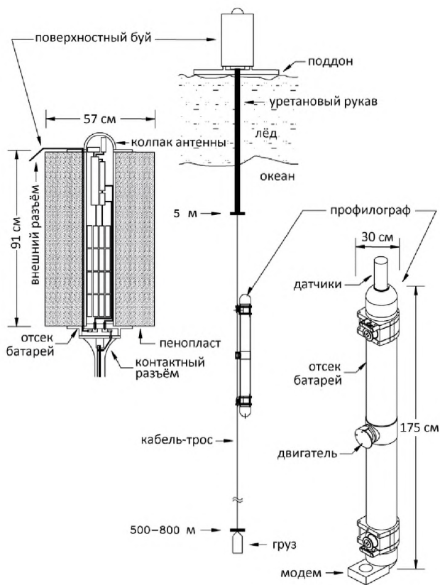
Рис. 17.13 Схема установки элементов комплекса ИТР
