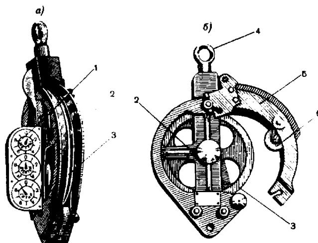
Рис. 6.82 Блок-счетчик 017
