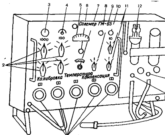
Рис. 11.2 Электросолемер ГМ-65
