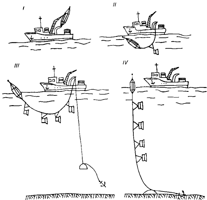
Рис.17.3 Схема постановки АБС комбинированным методом.
