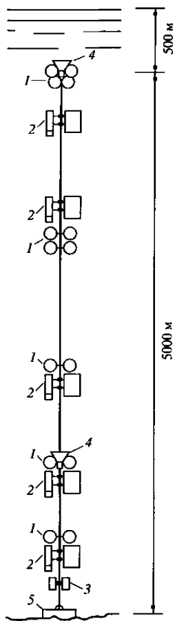
Рис. 17.5 Глубоководная автономная буйковая станция с распределенными плавучестями.
