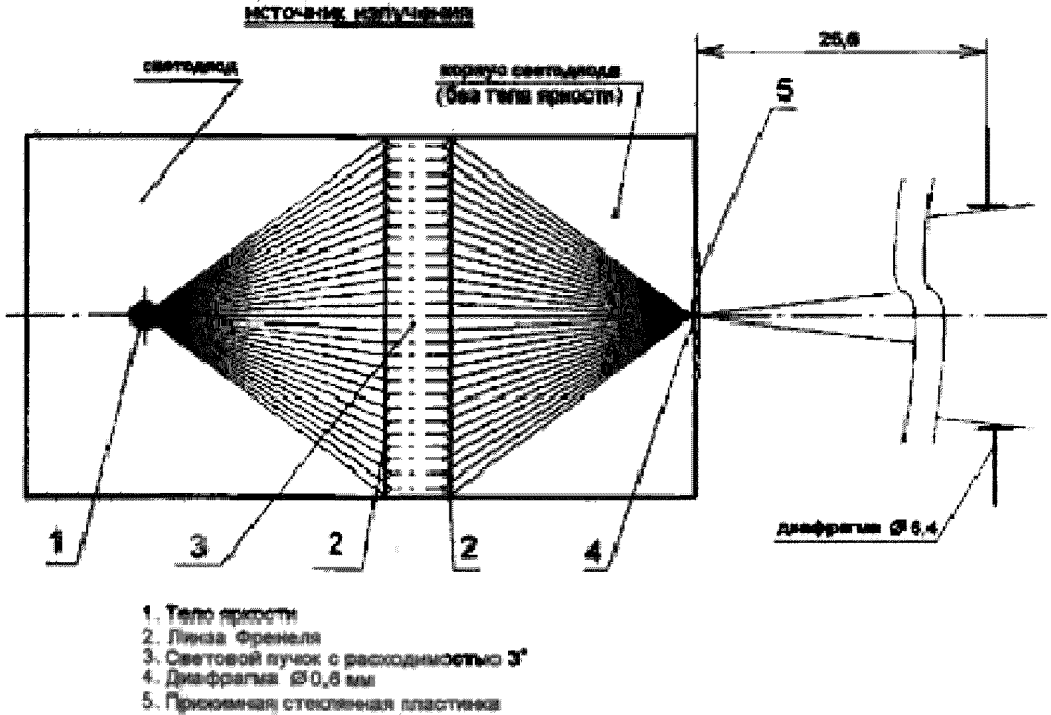
Рис.14.14 Оптическая схема источника излучения (пояснения в тексте)
