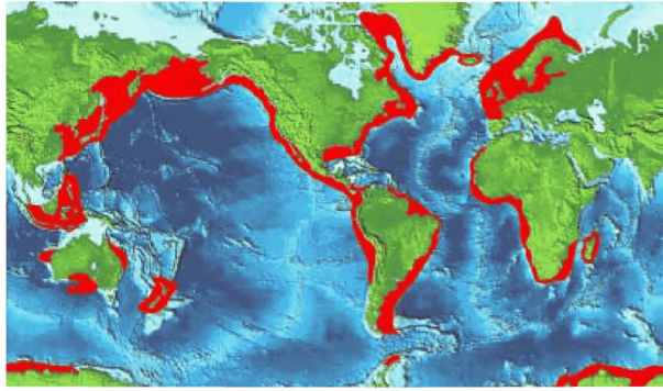
Рис. 16.7 Зоны апвеллинга Мирового океана
