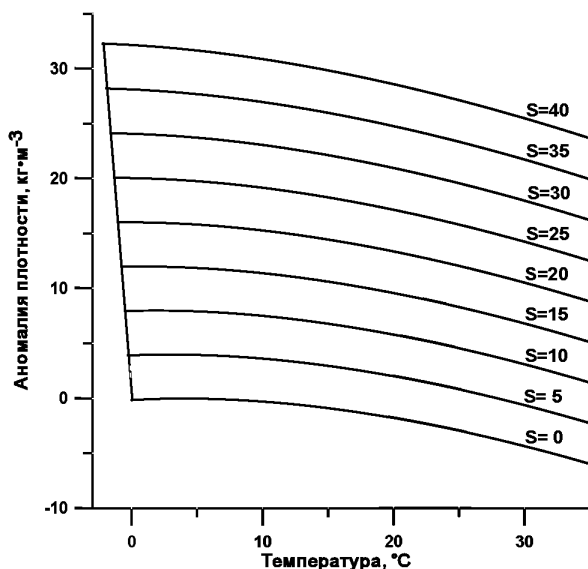
Рис.10.4 Аномалия плотности морской воды как функция от температуры и солёности при атмосферном давлении
