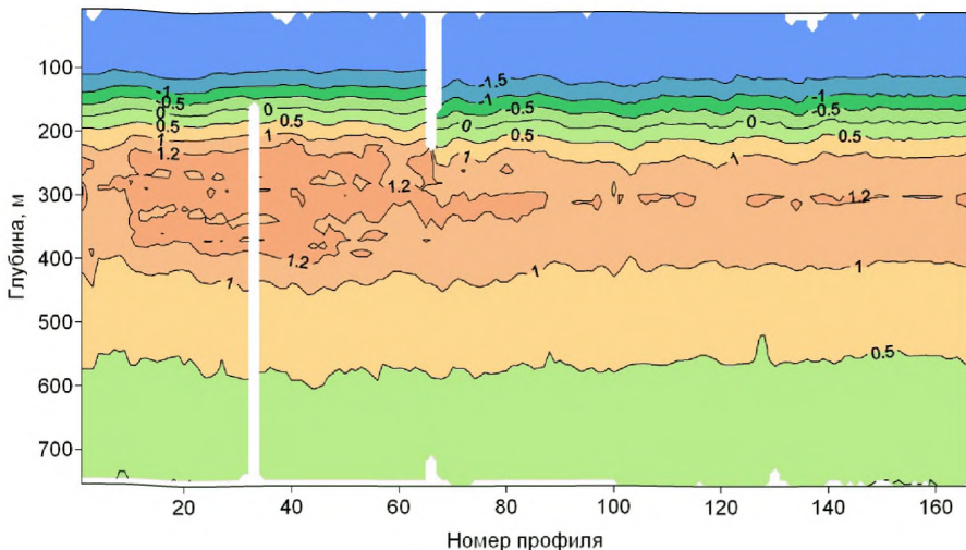
Рис. 17.15 Пример записи временной эволюции вертикального профиля температуры в приполюсном районе по данным ГТР-боя №14 в период с 13 сентября по 5 ноября 2007 г.
