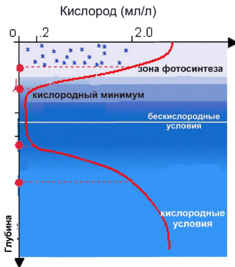
Рис. 16.6 Схематическое распределение растворенного кислорода по глубине
