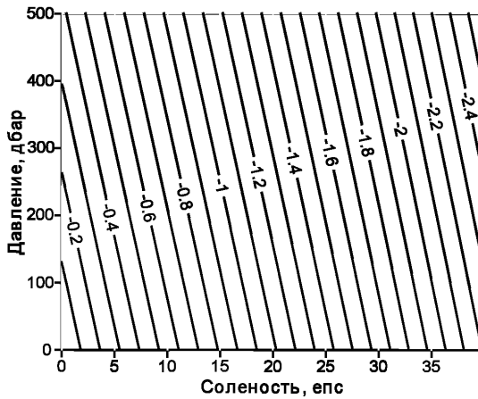
Рис. 10.1 Зависимость температуры замерзания морской воды ( ^\circ\text{C} ) от солености и давления.
