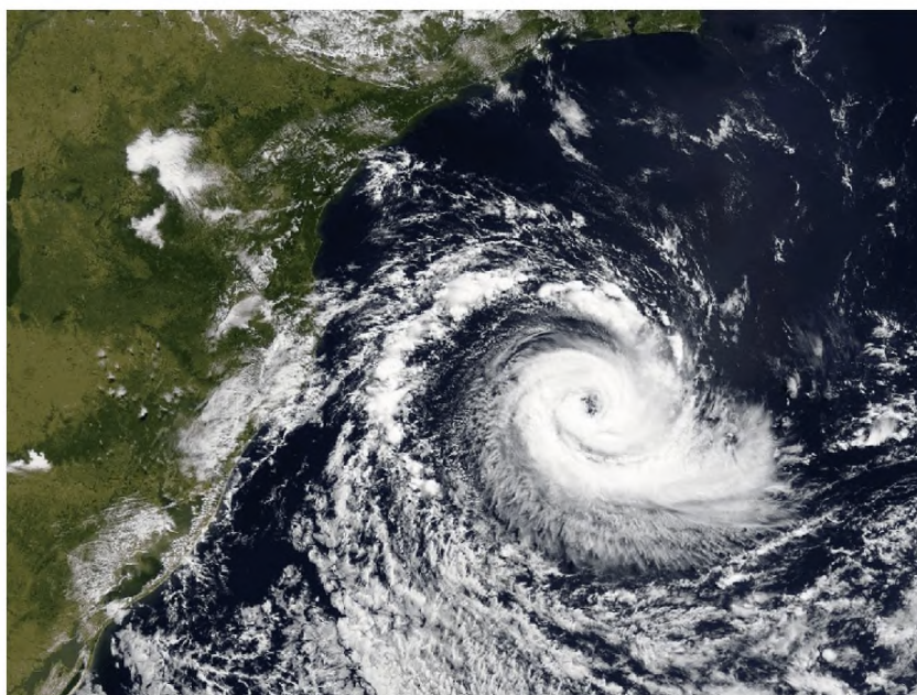
Рис.18.3 Тропический циклон, зарегистрированный спутниковым сканером MODIS к юго-востоку от побережья Бразилии 26 марта 2004 г.
