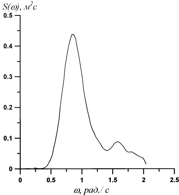
Рис.13.3 Энергетический спектр пульсаций давления
