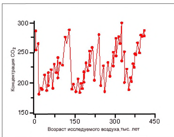
Рис. 16.5 Концентрация \text{CO}_2 в атмосфере по данным изучения ледового керна (Антарктида, станция «Восток»)
