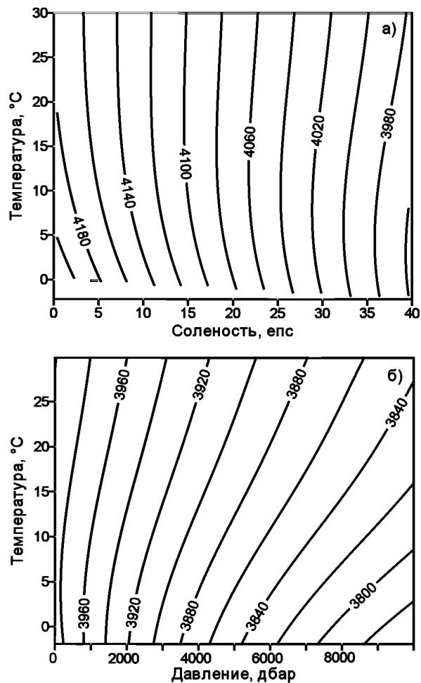
Рис. 10.3 Зависимость удельной теплоемкости при постоянном давлении c_p ( \text{Дж} \cdot \text{кг}^{-1} \cdot \text{°K}^{-1} ) от солёности и температуры при атмосферном давлении (а), давления и температуры при S = 35\text{‰} (б).
