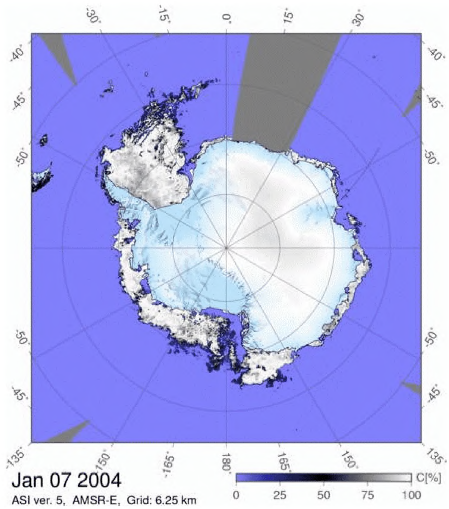
Рис. 18.6 Ледовая обстановка в Антарктике 7 января 2004 г. по данным СВЧ-радиометра AMSR-E
