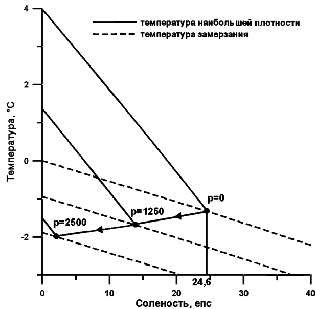
Рис. 10.2 Зависимость температуры наибольшей плотности и температуры замерзания морской воды ( ^{\circ}\text{C} ) от солёности ( \text{‰} ) и давления (дбар)
