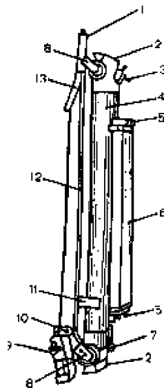
Рис. 7.13 Батометр морской БМ-48
