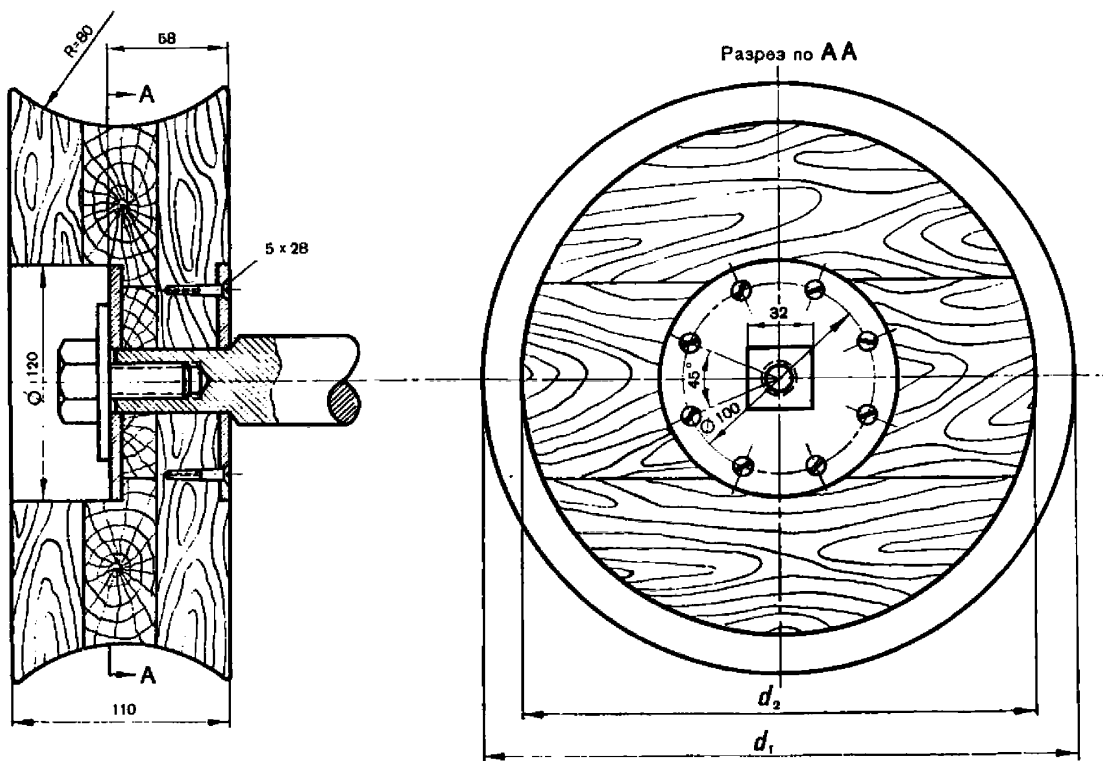
Рис. 6.74 Кабельная турочка к лебедкам «Океан» и ЛЭРОК
