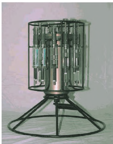
Рис. 7.11 Модель 1014 Syringe Sampler System , общий вид.
