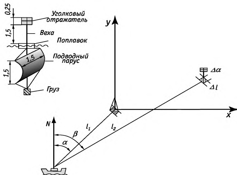
Рис. 12.1 Схема определения местоположения дрейфтера с помощью радиолокации в условной системе координат с началом в точке неподвижного ориентира. Заштрихованные области показывают возможную ошибку, на врезке дано схематическое изображение дрейфующего буя (все размеры в метрах).
