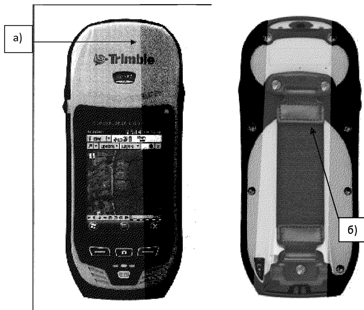
Рис.1.6 Внешний вид аппаратуры Trimble GeoExplorer 6000XH/6000XT а) место нанесения наклейки со знаком утверждения типа; б) место пломбировки.
