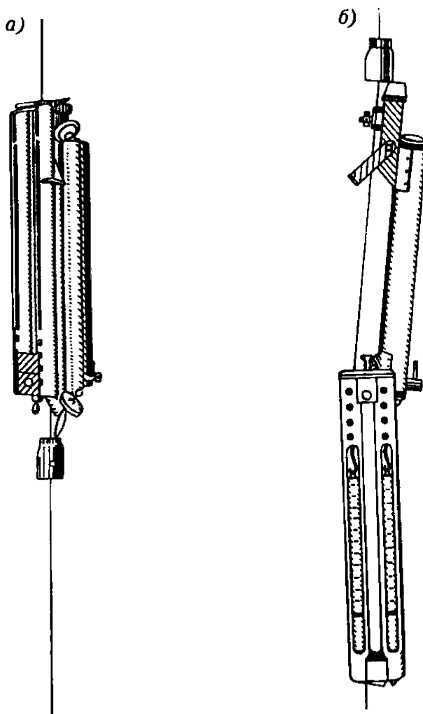
Рис. 7.18 Морской батометр системы ААНИИ в двух положениях:
