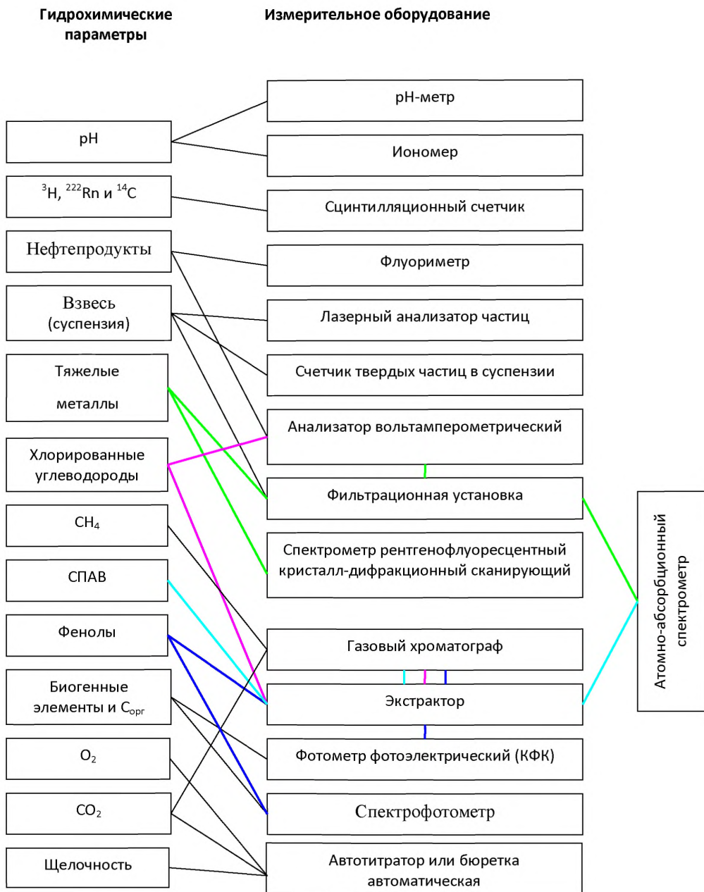
Рис. 16.14 Система приборов судовой гидрохимической лаборатории
