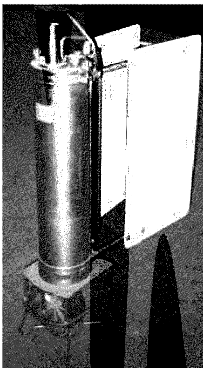
Рис. 12.7 Базовая модель измерителя течений и температуры «Поток-3».
