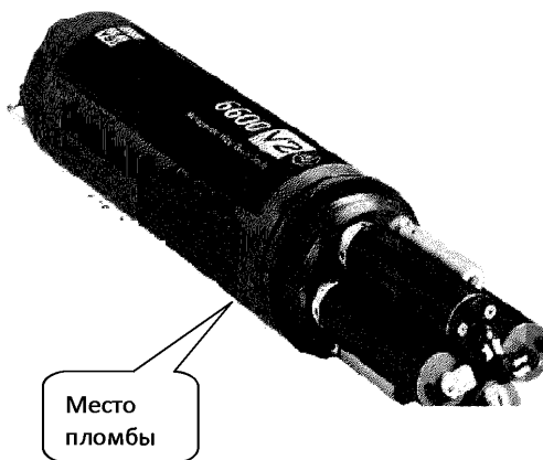
Рис.9.2 Внешний вид зонда гидрологического YSI 6600
