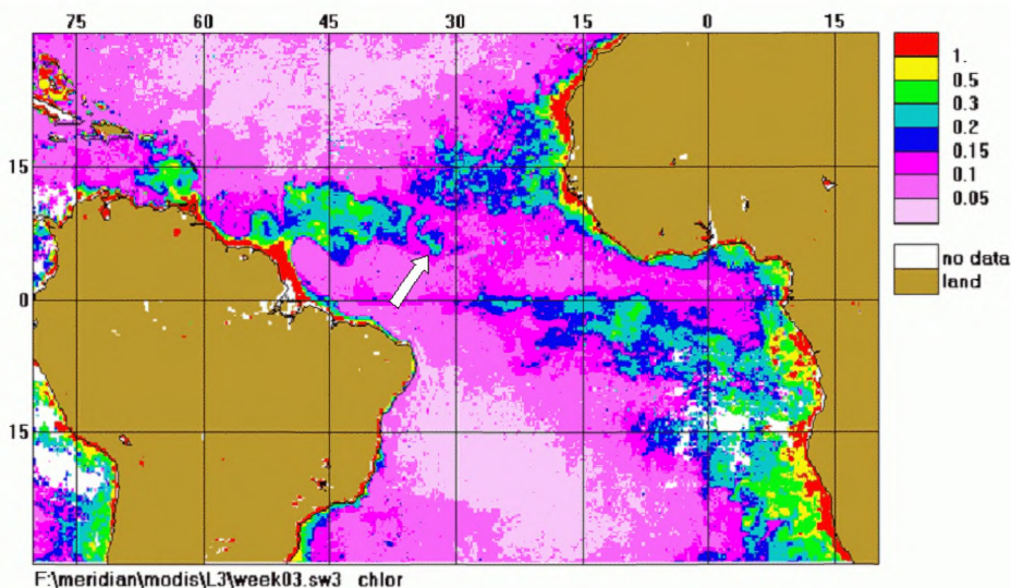
Рис. 19.6 Усредненное распределение концентрации хлорофилла в поверхностном слое океана, \text{mg}/\text{m}^3 , по данным сканера MODIS. Стрелкой указано положение линзы трансформированных амазонских вод. Изображение получено на борту НИС «Академик Сергей Вавилов» с ftp Лаборатории оптики океана ИОРАН с помощью спутникового терминала.
