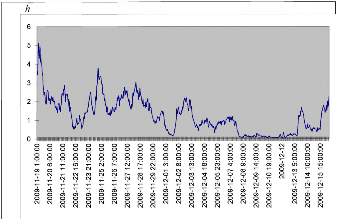
Рис. 13.4 Временной ряд средних высот волн
