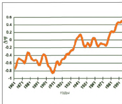
Рис. 16.1 Глобальные изменения температуры (1861-1996 г.)
