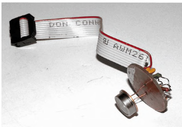
Рис.14.11 Фотодиод с прецизионным усилителем
