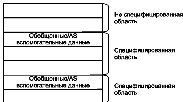
Рисунок 39 — Обобщенная структура блока составных данных
