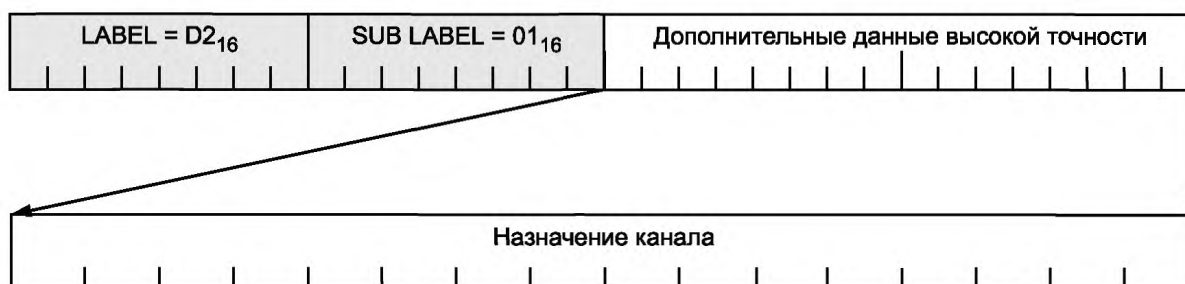
Рисунок 48 — Вспомогательные данные с назначением каналов высокой точности
