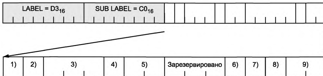
Рисунок 66 — Вспомогательные данные для CCI
