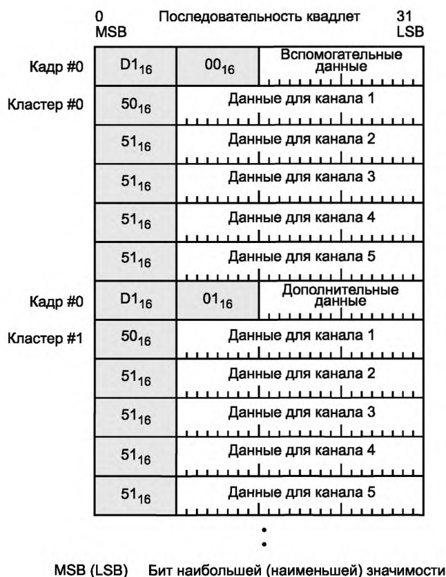
Рисунок 63 — Пример потока SACD в случае пяти каналов
