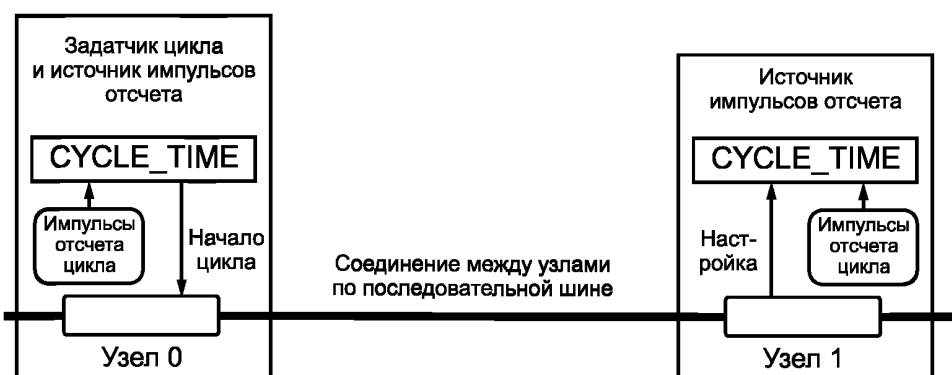
Рисунок С.1 — Шина с двумя узлами
