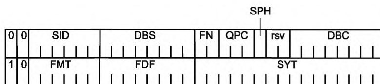
Рисунок 5 — Формат общего изохронного пакета (CIP)
