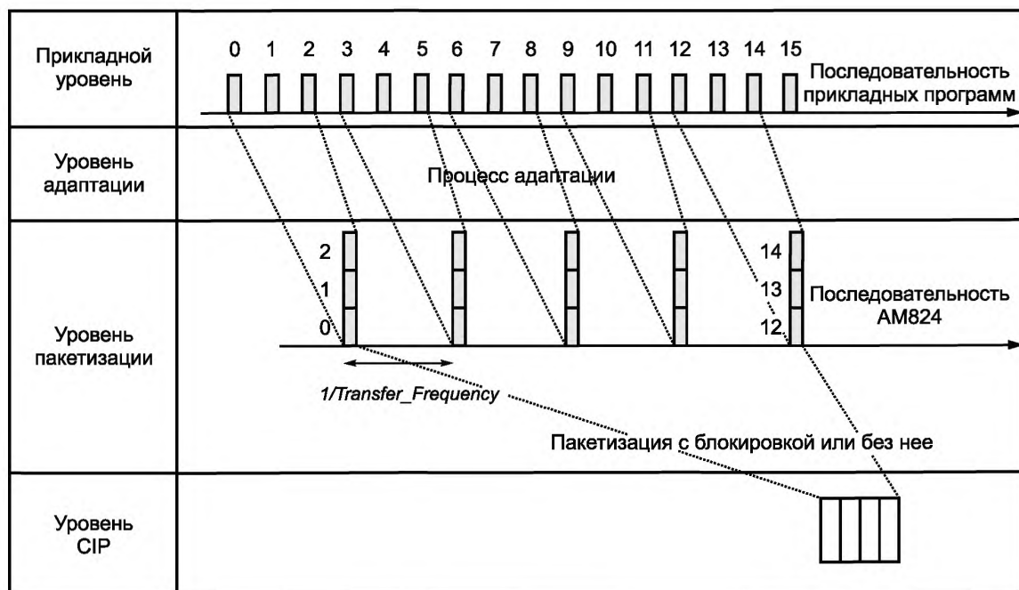
Рисунок 35 — Адаптация к последовательности AM824
