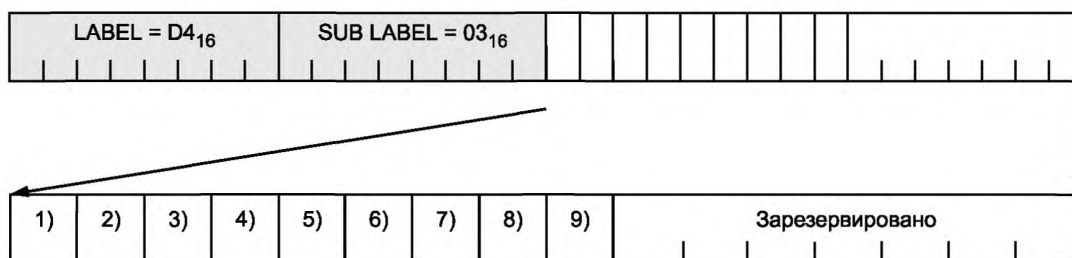
Рисунок 77 — Данные, передаваемые в каждом блоке данных группы 3 для фиксированной канальной структуры
