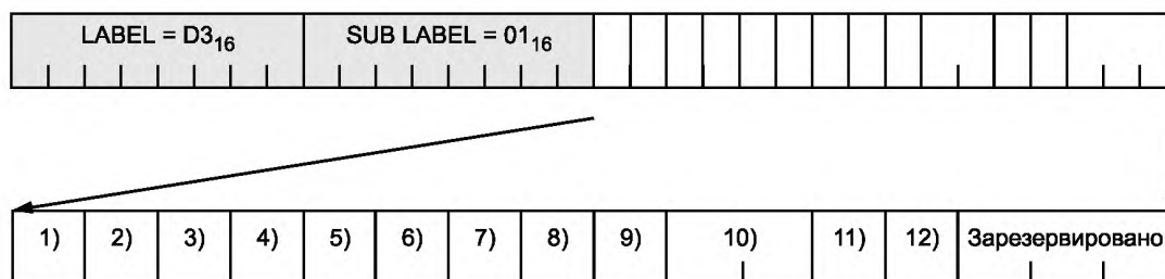
Рисунок 65 — Данные, передаваемые в каждом блоке данных
