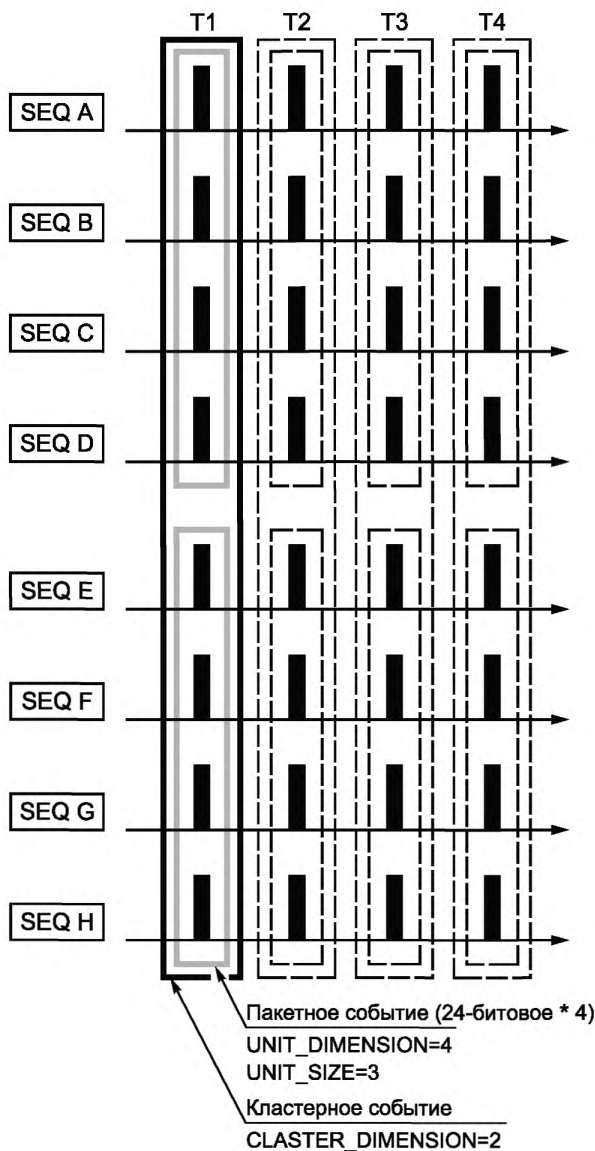
Рисунок 10 — Пакетные и кластерные события
