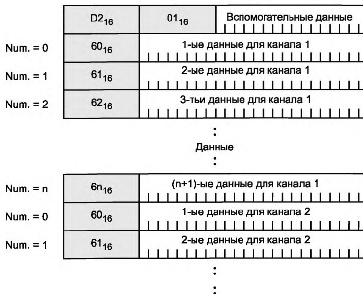
Рисунок 22 — Обобщенная последовательность квадлет высокой точности
