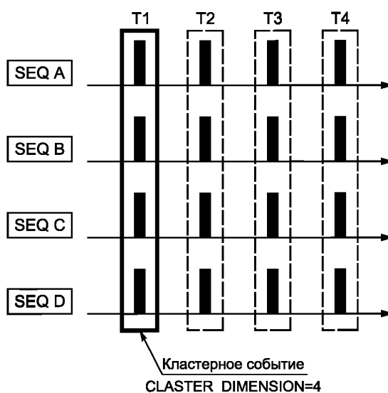
Рисунок 9 — Кластерные события
