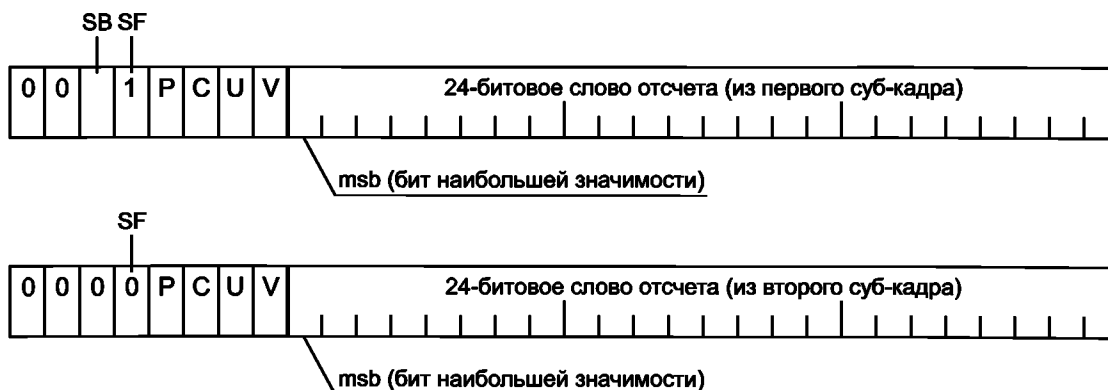
Рисунок 15 — Формат данных, совместимый с МЭК 60958
