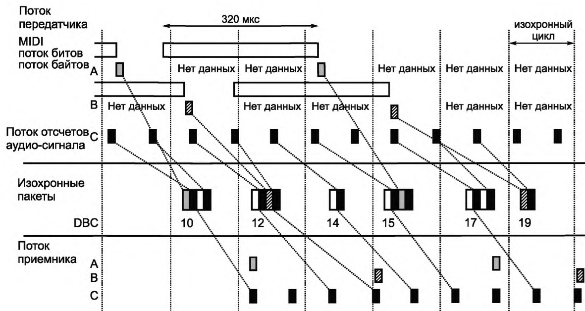
Рисунок 44 — Мультиплексирование потоков данных MIDI
