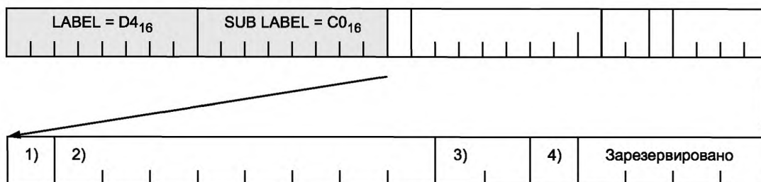
Рисунок 82 — Вспомогательные данные для CCI
