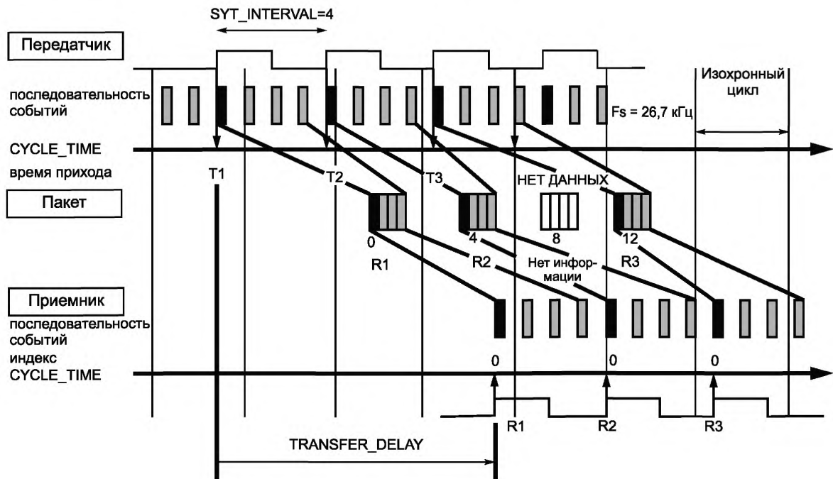
Рисунок 8 — Метод передачи с блокировкой
