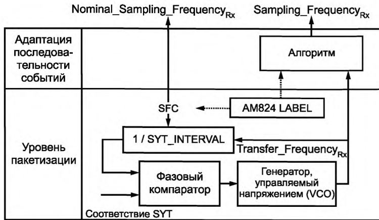
Рисунок 3 — Пример реализации приемника
