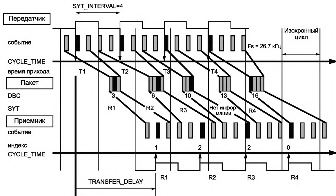
Рисунок 6 — Метод передачи без блокировки
