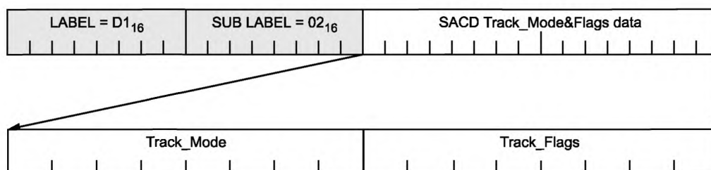
Рисунок 60 — Данные Track_Mode&Flags SACD
