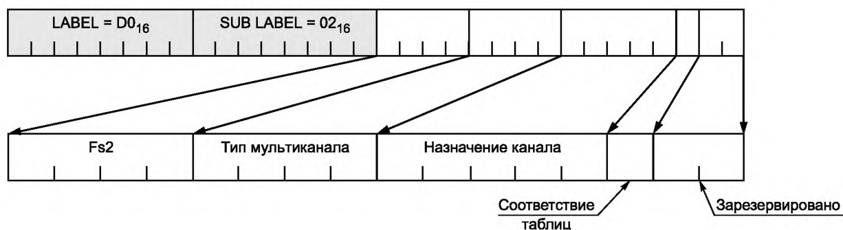
Рисунок 52 — Данные, передаваемые в точке начала данных
