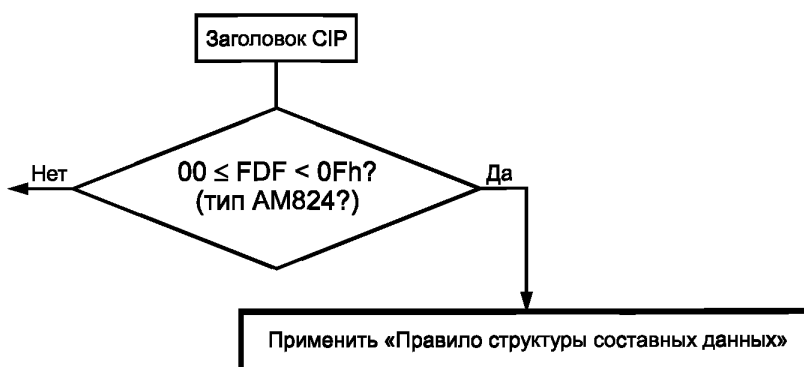
Рисунок 38 — Условие применения правила AM824
