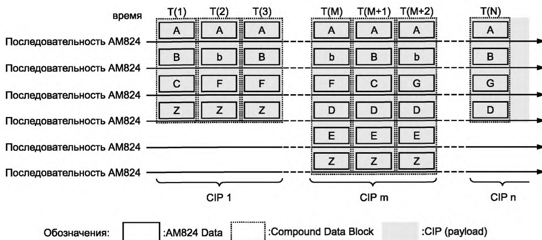
Рисунок 37 — Пример использования блока составных данных
