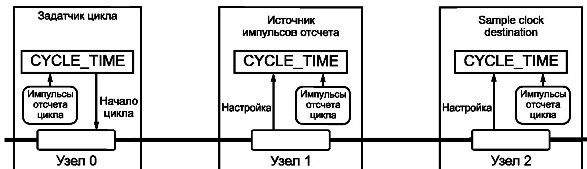
Рисунок С.2 — Шина с тремя узлами
