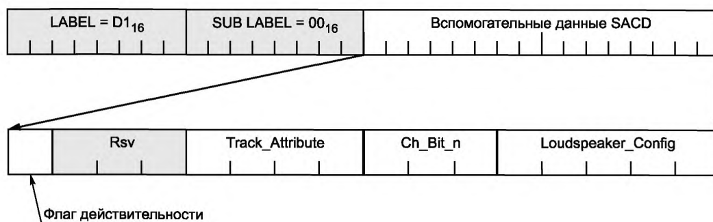
Рисунок 58 — Вспомогательные данные SACD
