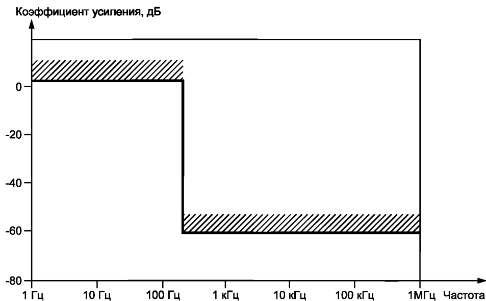
Рисунок С.4 — Образец затухания джиттера при восстановлении импульсов отсчетов
