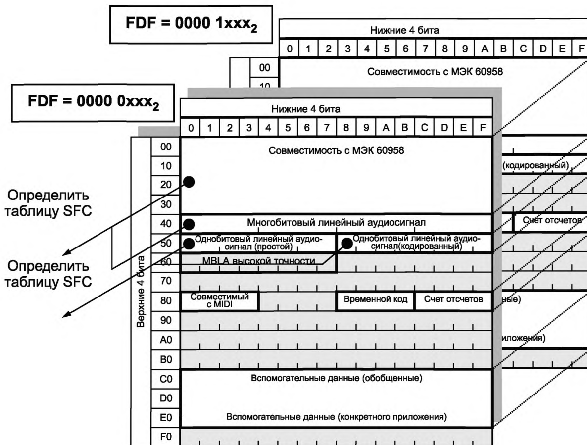
Рисунок 34 — FDF для AM824 и пространство LABEL AM824
