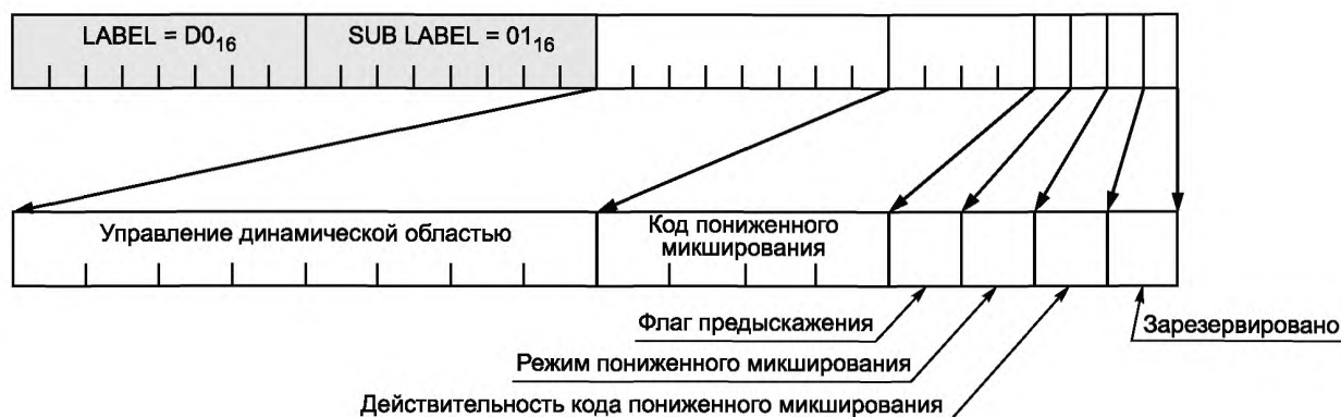
Рисунок 53 — Данные, передаваемые в каждом блоке данных
