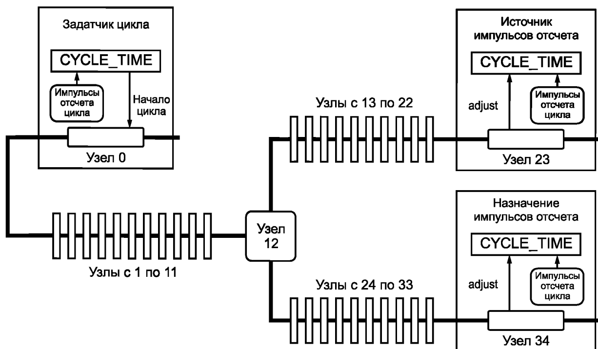
Рисунок С.3 — Шина с тридцатью пятью узлами
