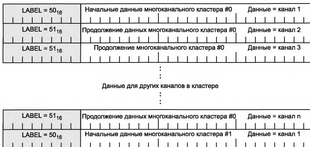
Рисунок 42 — Обобщенная последовательность квадлетов однобитового аудиосигнала.
