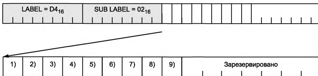
Рисунок 76 — Данные, передаваемые в каждом блоке данных группы 2 для фиксированной канальной структуры
