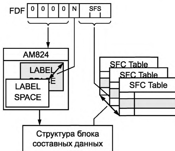
Рисунок 33 — Интерпретация SFC
