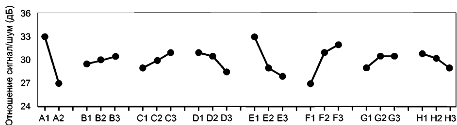
Рисунок 4 — Диаграмма факторных эффектов для отношения SN (робастность)
