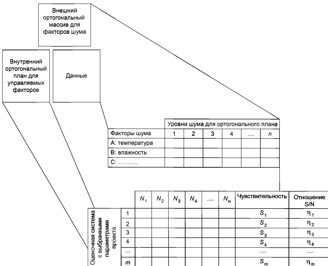
Рисунок 3 — План прямого производства для параметрического планирования
