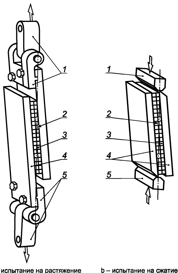
а – испытание на растяжение
