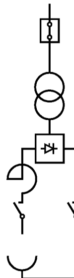
Рисунок АА.5 — Источник постоянного тока печи с высоковольтным переключателем (или высоковольтным выключателем печи) в закрытом положении, клапанные импульсы запуска остановлены, и переключатель низковольтного разъединителя в открытом положении
