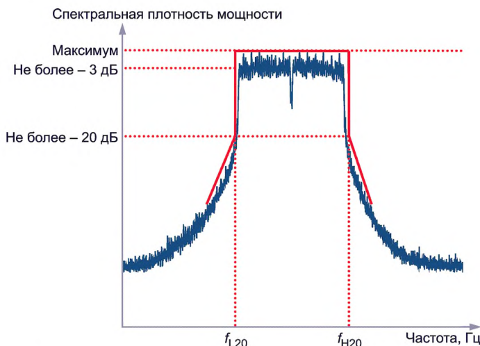
Рисунок 10 — Частоты среза, полученные от максимального уровня мощности
