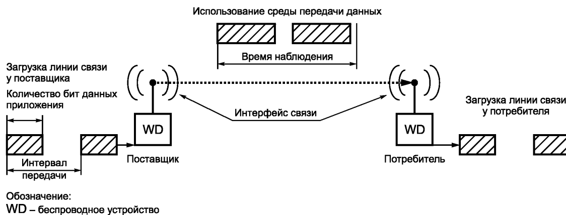
Рисунок 8 — Загрузка линии связи при наличии двух беспроводных устройств
