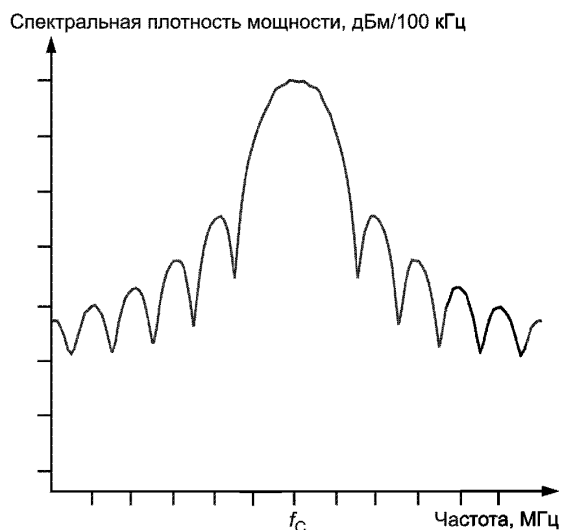
Рисунок 15 — Спектральная плотность мощности системы IEEE 802.15.4
