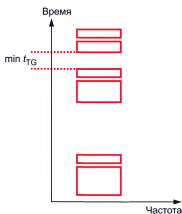
Рисунок 16 — Минимальный обрыв (пауза) передачи сигнала
