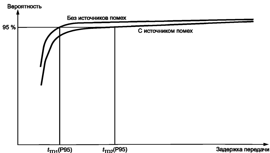
Рисунок 19 — Пример функций распределения времени передачи
