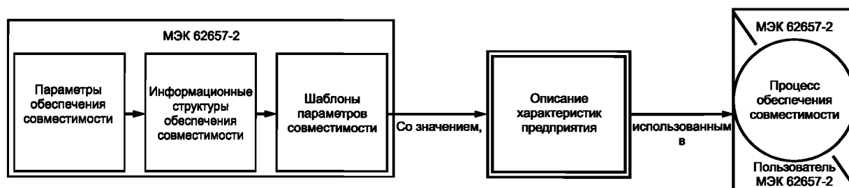
Рисунок 23 — Параметры для описания общей заводской характеристики
