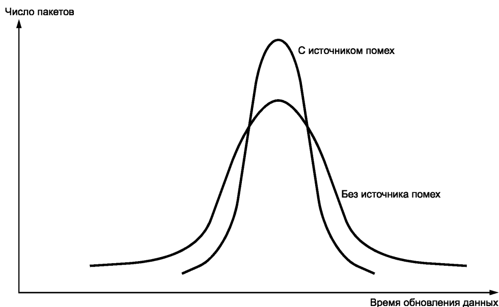
Рисунок 21 — Пример функций распределения времени обновления данных
