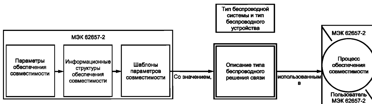
Рисунок 28 — Параметры для описания решения беспроводной связи
