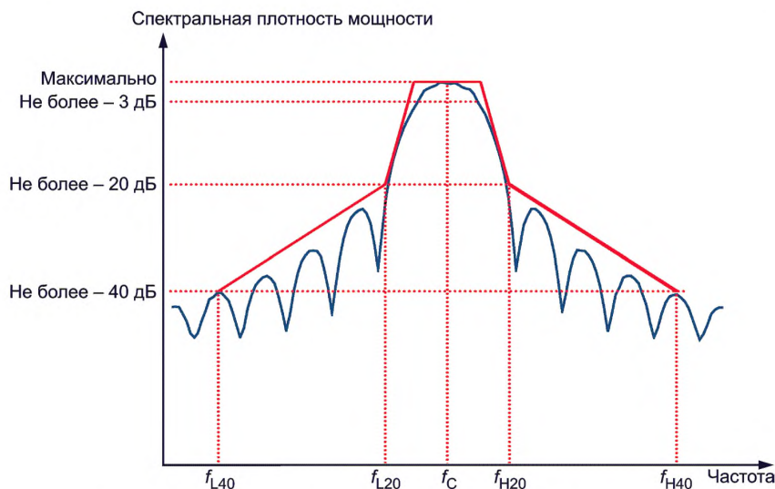
Рисунок 20 — Спектральная маска передатчика системы IEEE 802.15.4
