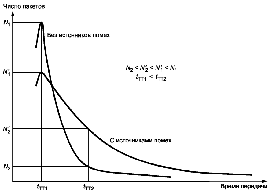
Рисунок 18 — Пример функций плотности распределения времени передачи
