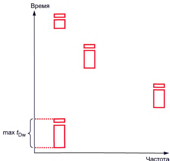
Рисунок 12 — Максимальное время выдержки
