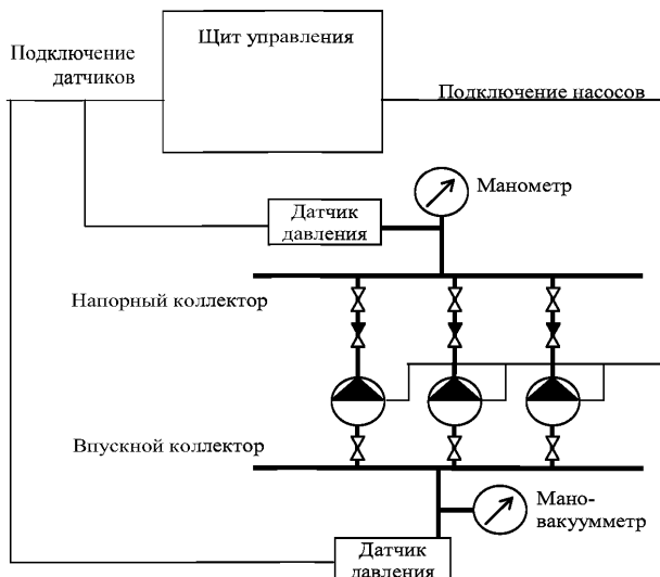
Рисунок 4.4 – Типовая структурная схема МАНС (на базе трех насосов)
