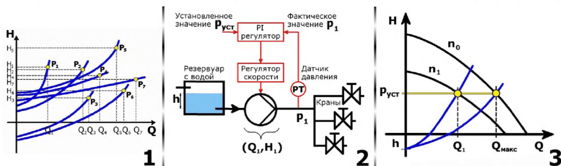
1 – изменчивость системы; 2 – общая схема; 3 – рабочие точки и характеристики
