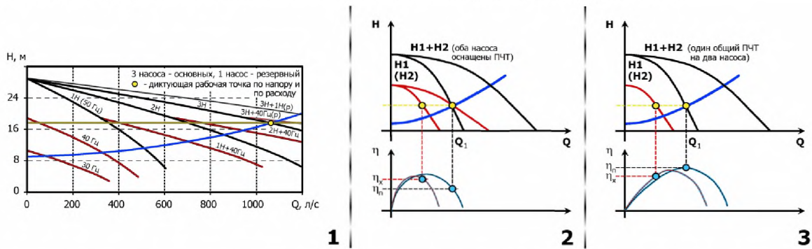
1 – регулирование по постоянному давлению; 2 – вариант КПД двух насосов, оснащенных ПЧТ; 3 – вариант КПД насоса в ПНУ (МАНС), оснащенной одним ПЧТ Рисунок В.6 – Графики параллельной работы насосов совместно с ЧРП
