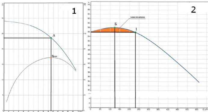
1 – стабильно нисходящая кривая; 2 – восходящая кривая
