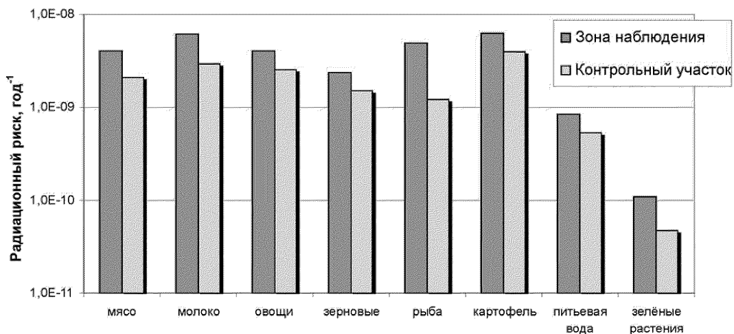
Рисунок Е.3 – Радиационный риск от потребления 137 Cs с отдельными продуктами питания и питьевой водой в зоне наблюдения БалАЭС и на контрольном участке (с. Маянга)
