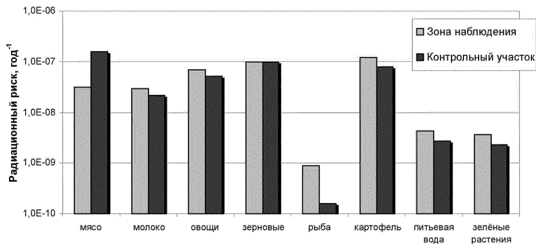
Рисунок Е.4 – Радиационный риск от потребления 90 Sr с отдельными продуктами питания в зоне наблюдения БалАЭС и на контрольном участке (с. Маянга)
