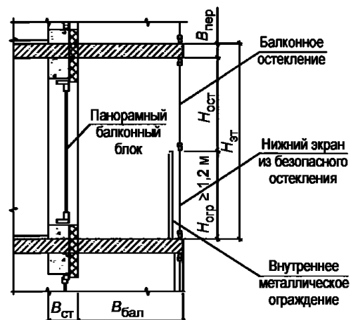
Принципиальная схема компоновки балкона (вариант с панорамным балконным блоком)
