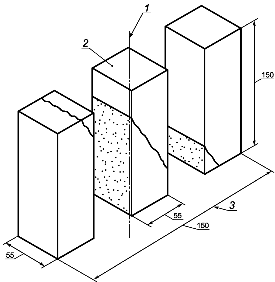
1 — главная ось; 2 — контрольный образец-призма; 3 — размер до распиливания плиты (заготовки)
