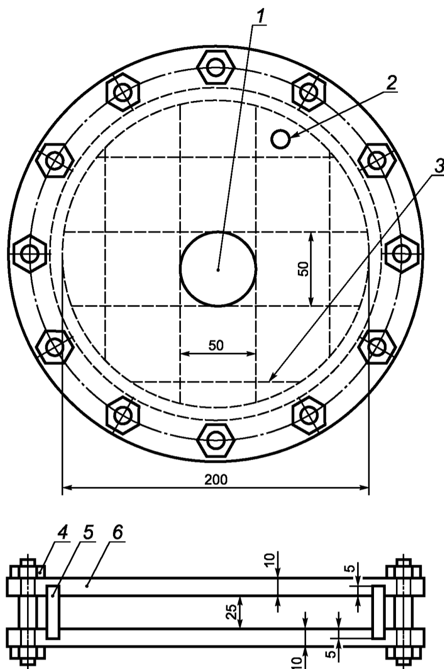
1 — отверстие для заполнения; 2 — отверстие с клапаном; 3 — линия разреза; 4 — болты М12 (12 шт.); 5 — стальное кольцо диаметром 200 мм; 6 — стальная пластина диаметром 270 мм
