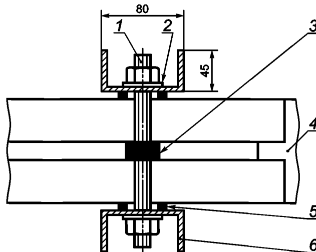
1 — шпилька резьбовая М10; 2 — шайба металлическая; 3 — прокладка для создания зазора между плитами; 4 — материал заделки контура зазора; 5 — шайба резиновая; 6 — траверса крепления
