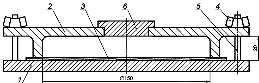
1 — плита основания; 2 — камера; 3 — образец; 4 — гайка-барашек; 5 — болт; 6 — пробка
