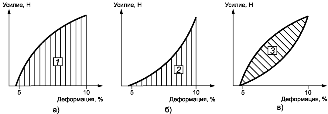
Рисунок С.3 — Работа цикла нагружение/разгружение
