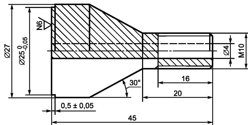
Рисунок М.2 — Конический штамп
