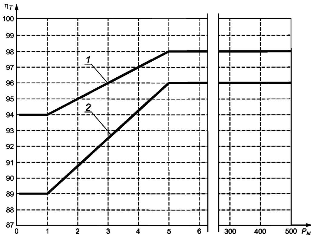
Рисунок В.2 — Задаваемые по умолчанию значения КПД для ременной передачи
