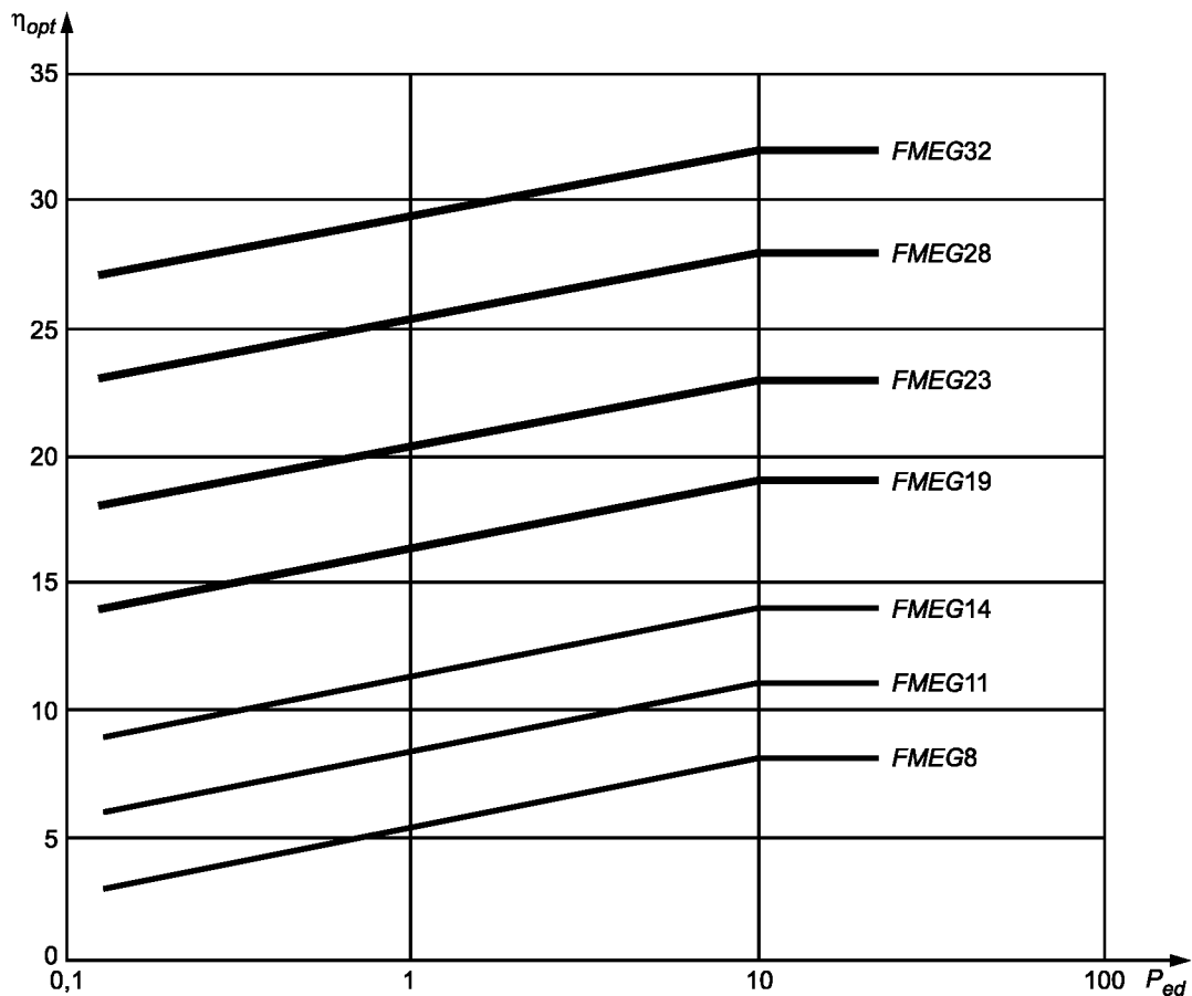
Рисунок 8 — Показатели эффективности диаметральных вентиляторов, имеющих привод
