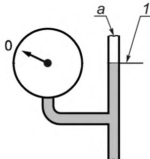
1 — эталонная плоскость манометра; a — открыто в атмосферу
