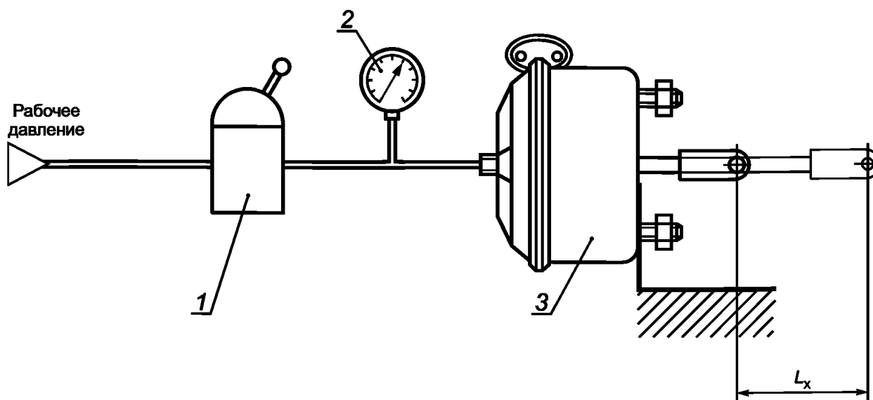
1 — кран точного регулирования; 2 — манометр; 3 — объект испытаний; L_x — ход штока
