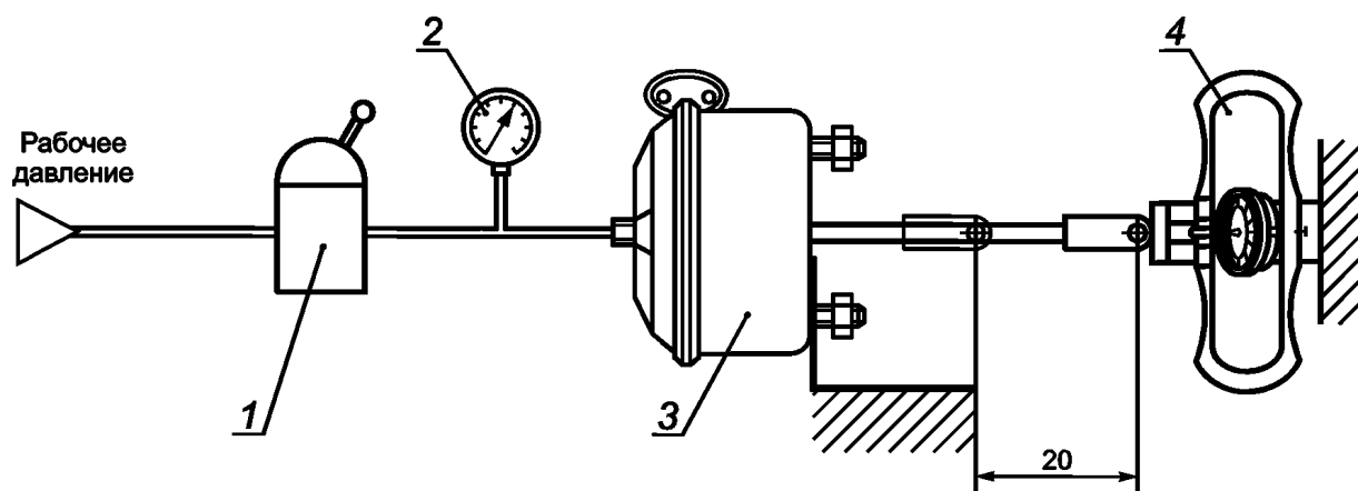
1 — кран точного регулирования; 2 — манометр; 3 — объект испытаний; 4 — динамометр сжатия
