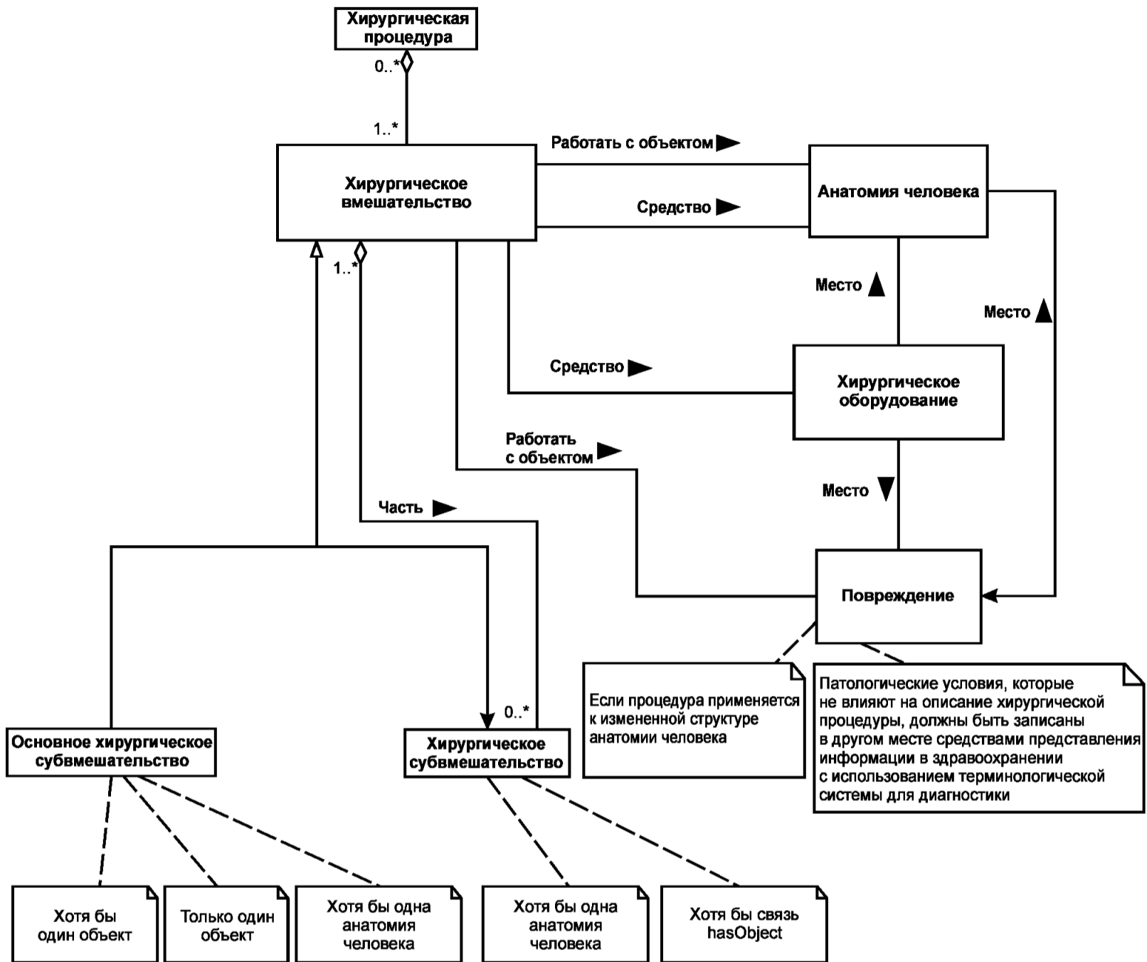
Рисунок 1 — UML диаграмма
